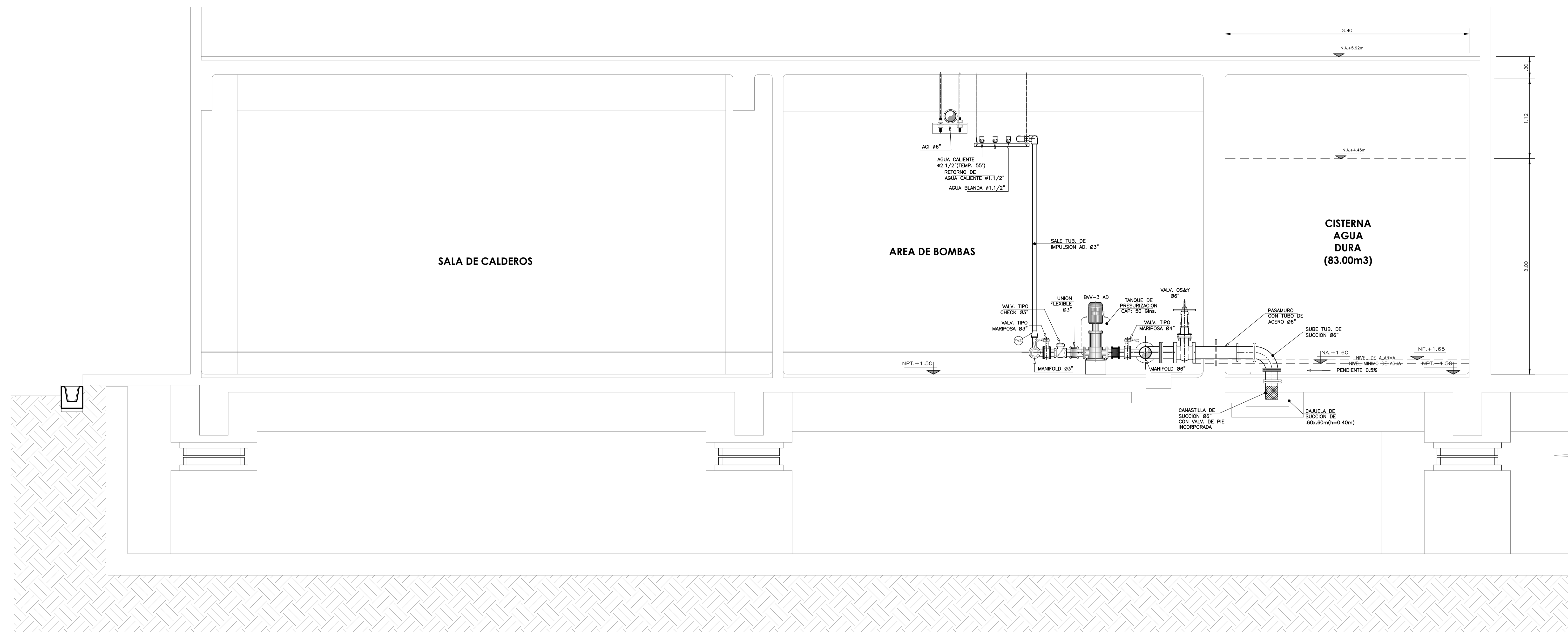
CORTE B - B ESCALA: 1/25
