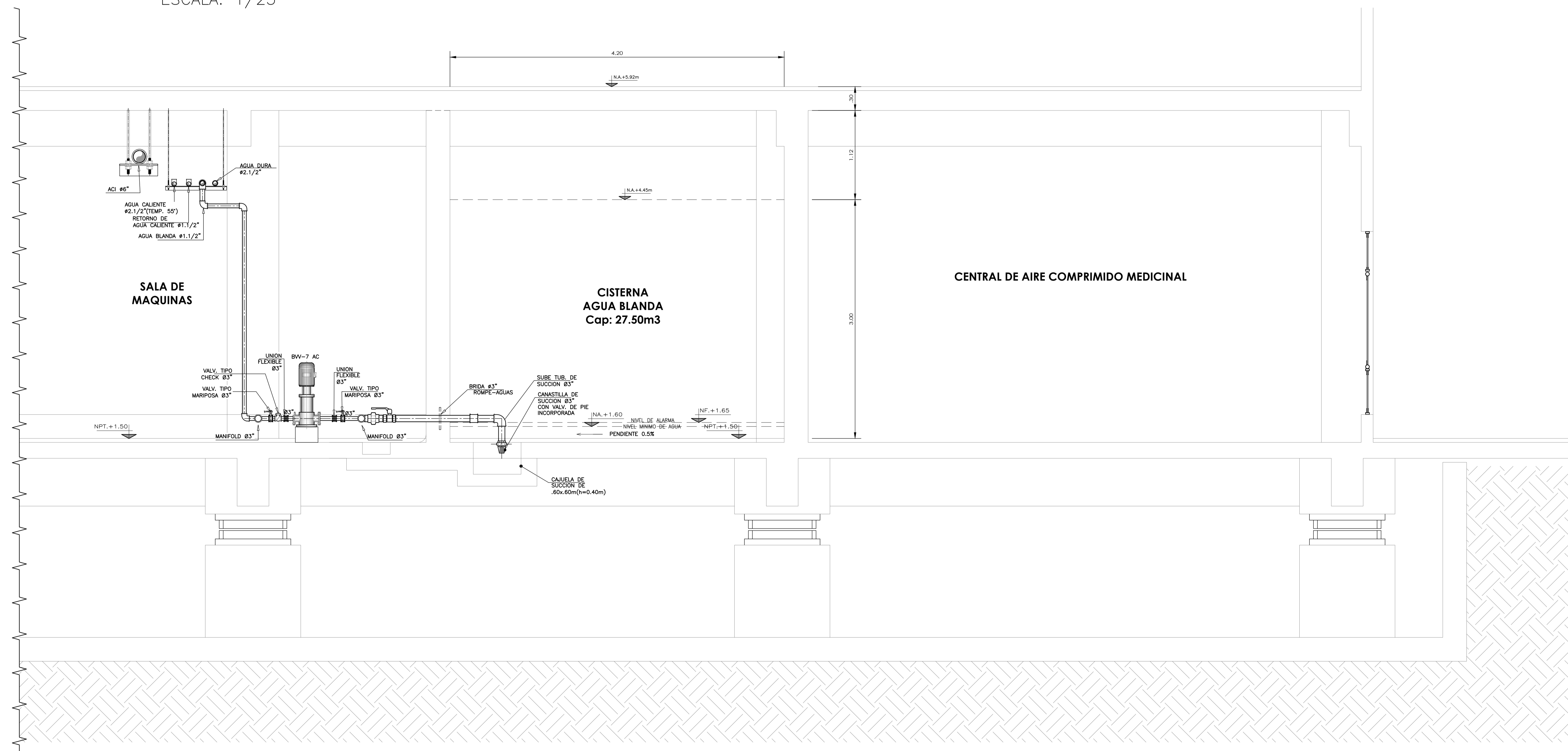
CORTE C - C ESCALA: 1/25
