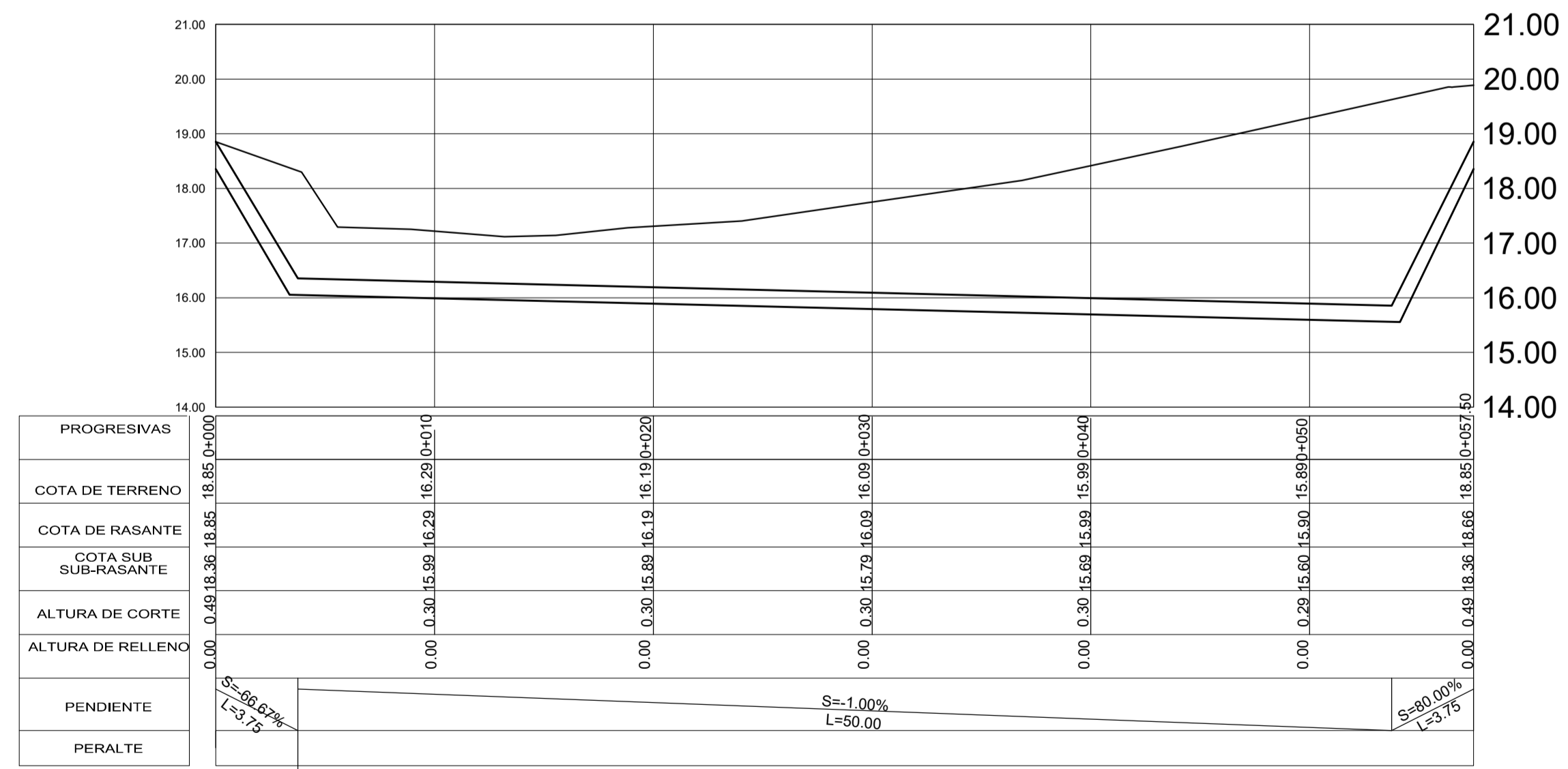
PERFIL LONGITUDINAL ESCALA HORIZONTAL: 1/200 ESCALA VERTICAL: 1/100
