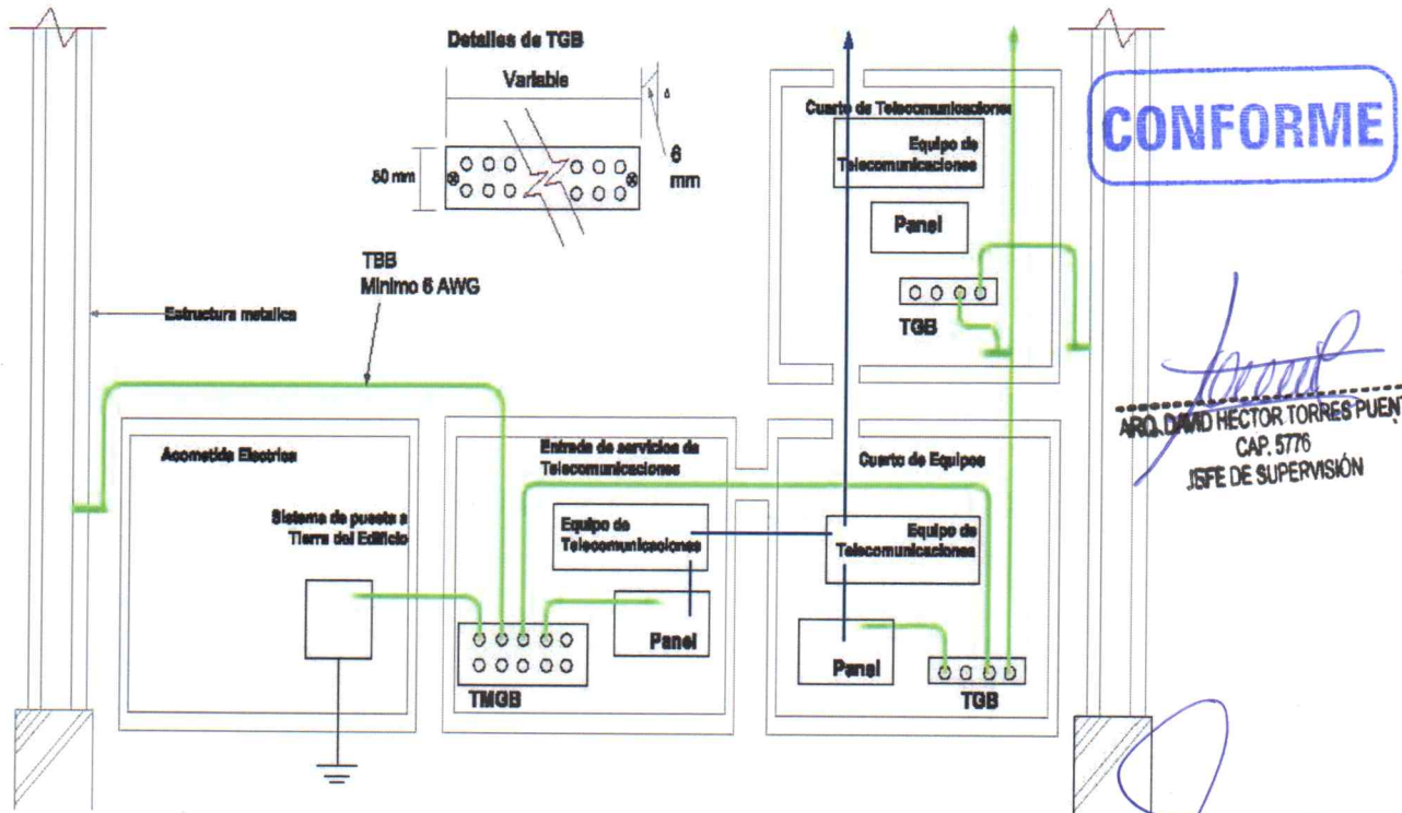
Fig. Esquema SPT comunicaciones
