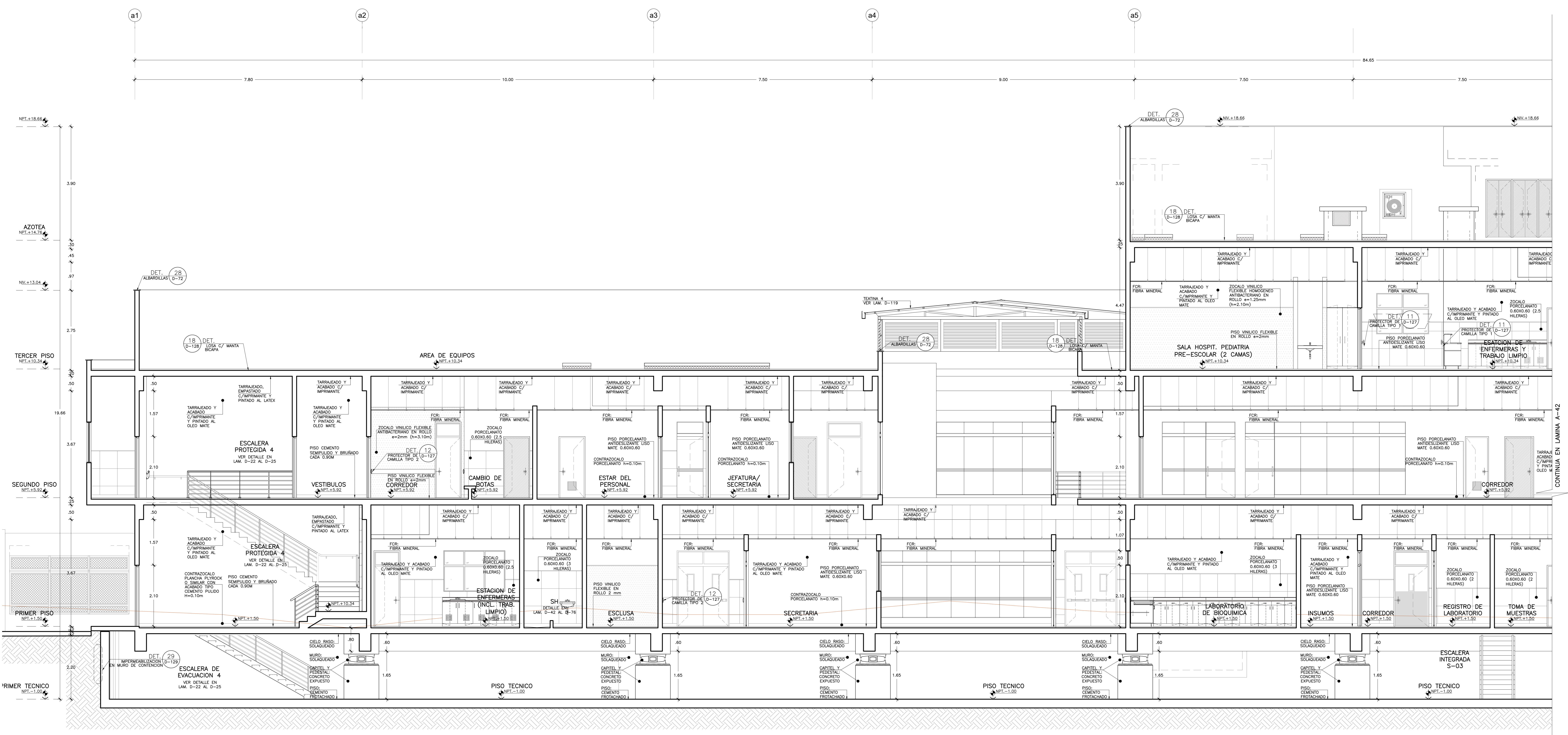
BLOQUE A CORTE B-B (SECTOR 1) Esc. 1:50
