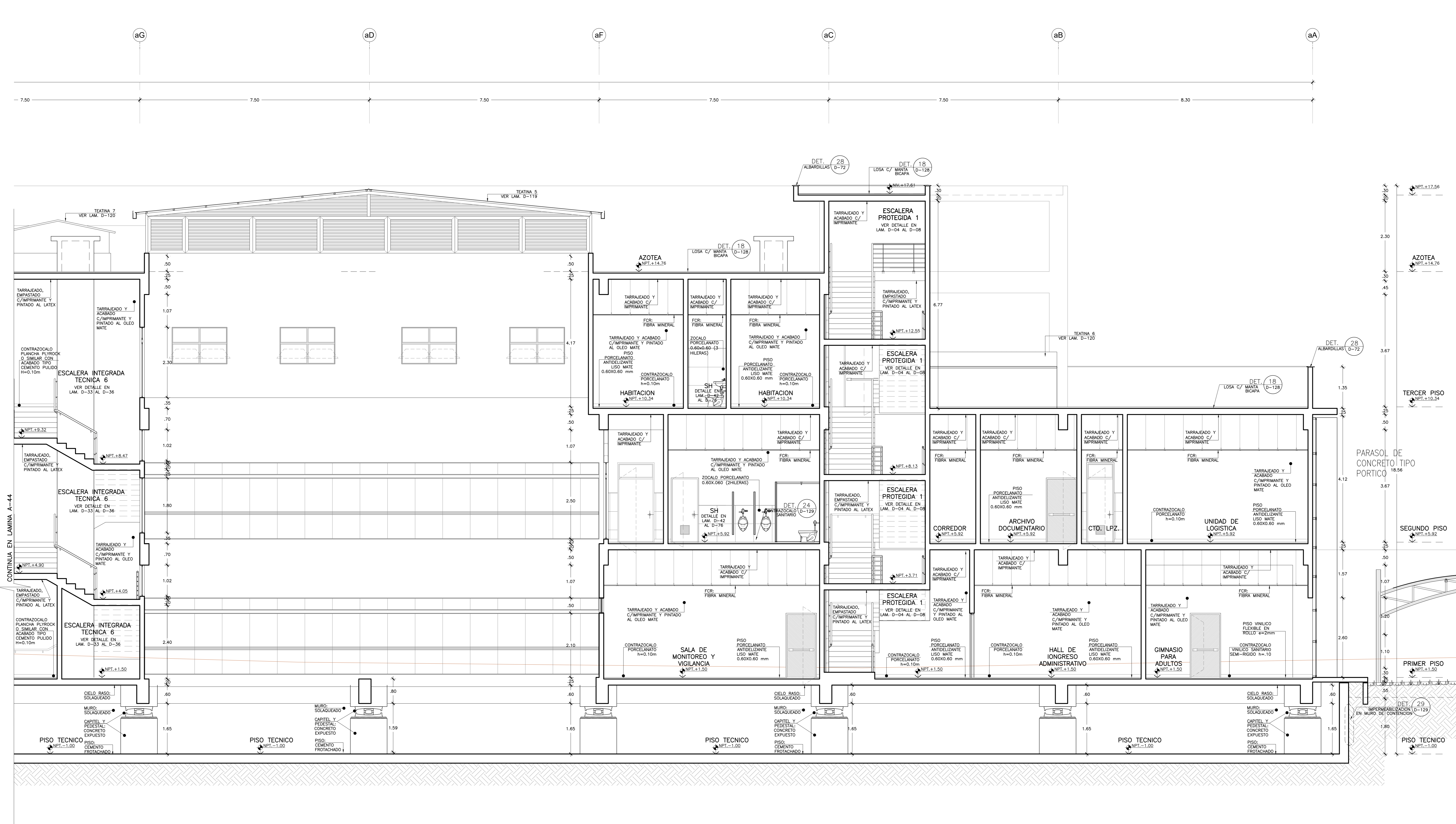
BLOQUE A CORTE C-C (SECTOR 3) Esc. 1:50
