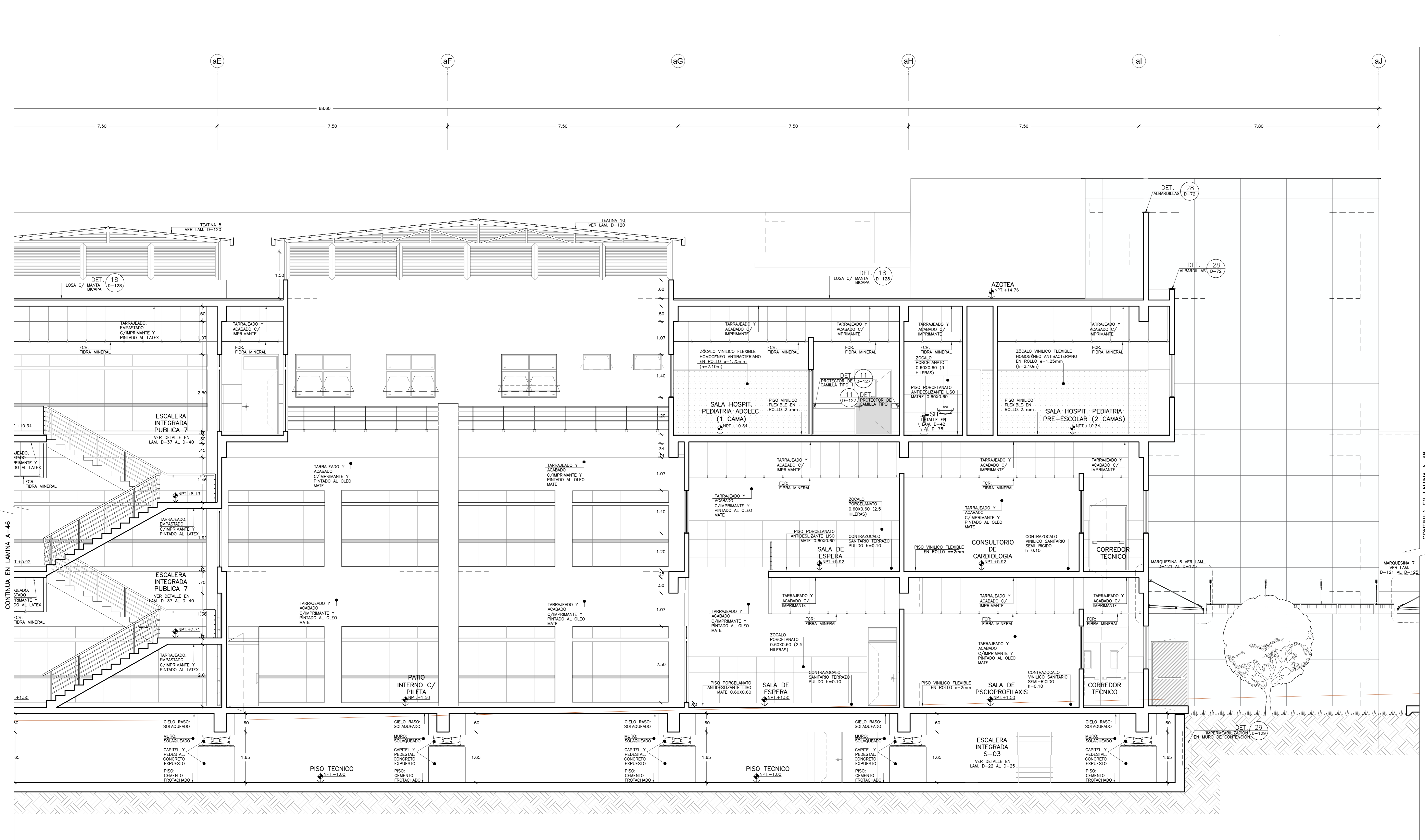
BLOQUE A CORTE D-D (SECTOR 2) Esc. 1:50
