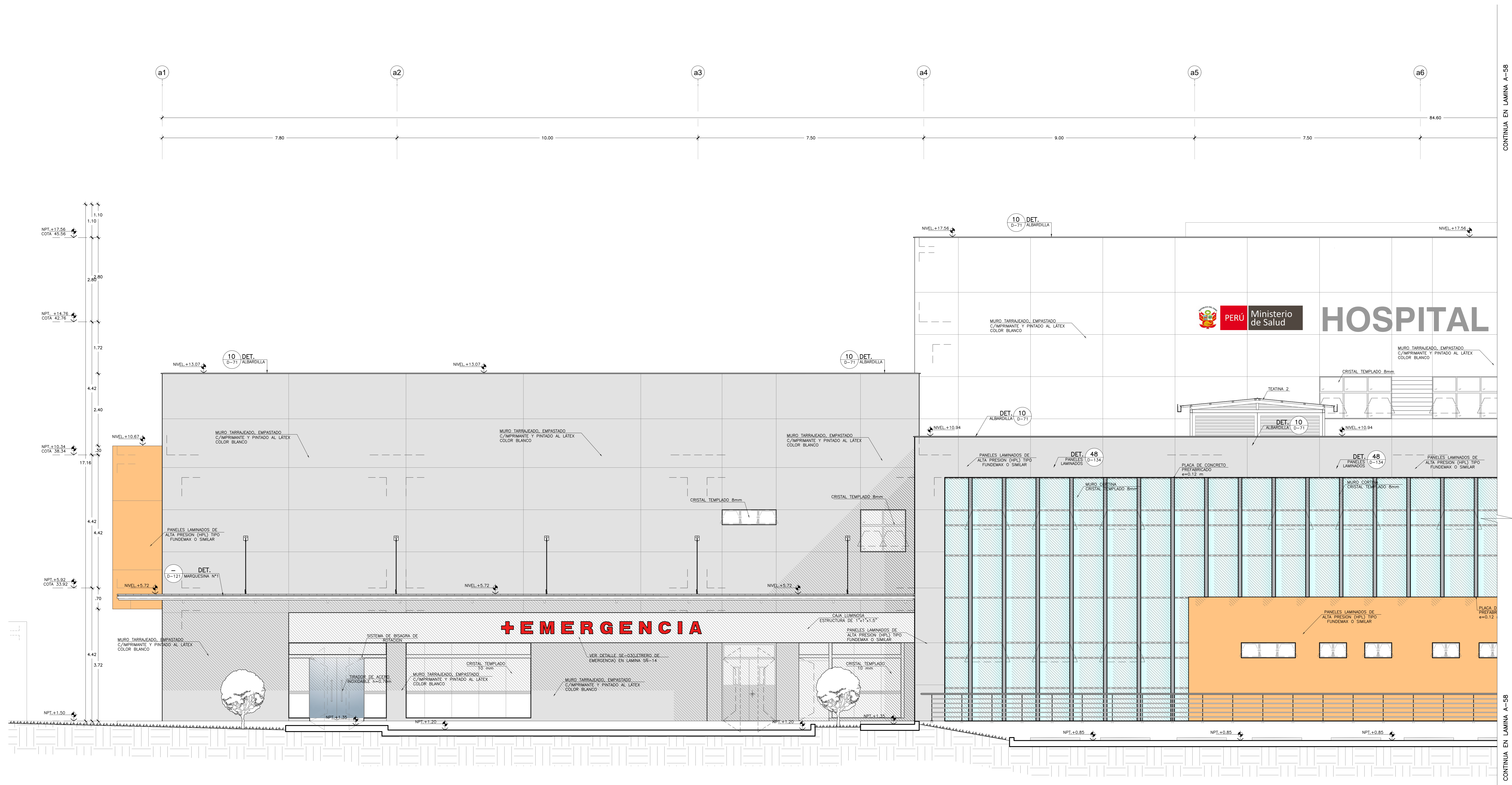
ELEVACION 1 SECTOR A Esc. 1:50
