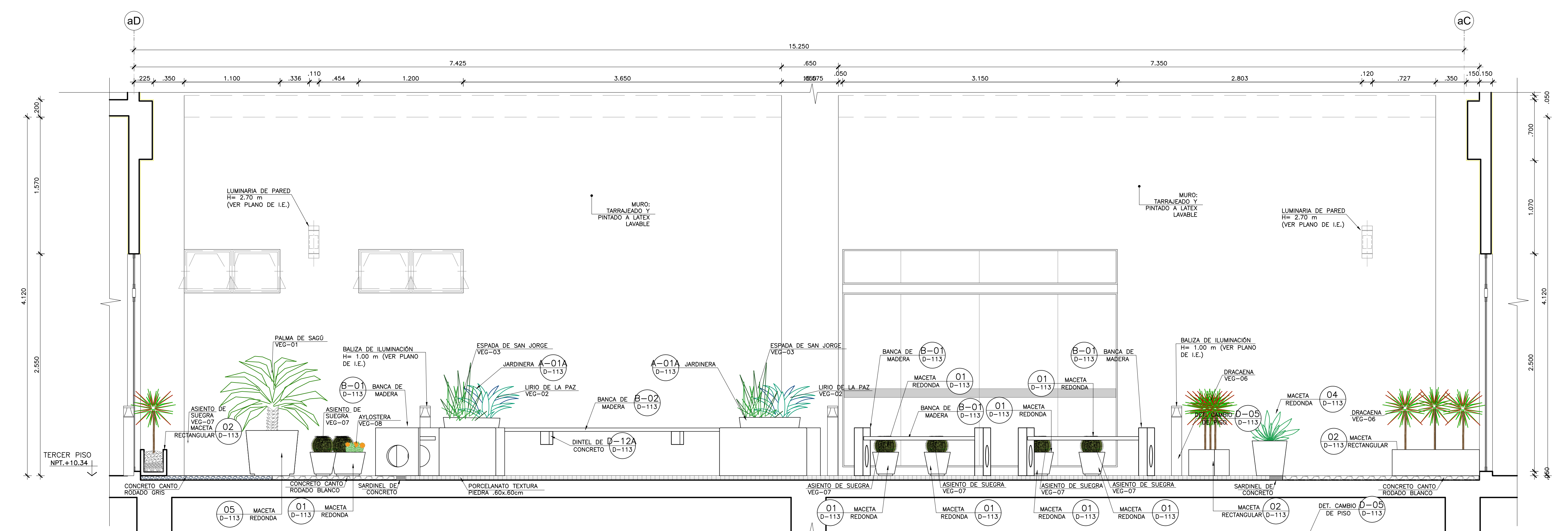
CORTE A-A' TERRAZA N°1 Esc. 1:25
