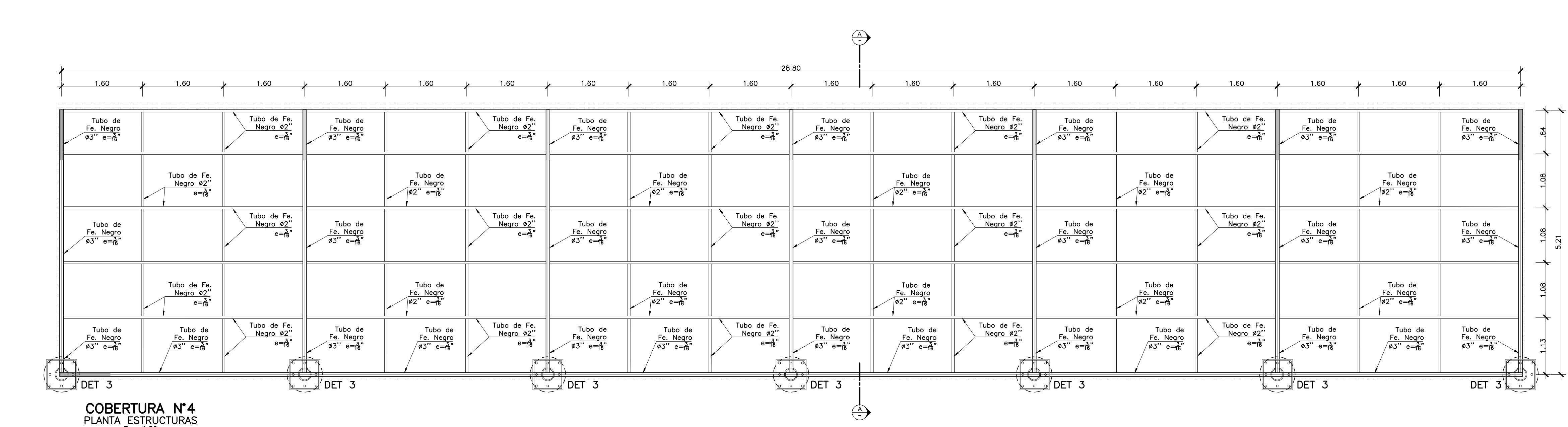
COBERTURA N°4 PLANTA ESTRUCTURAS Esc. 1:25
