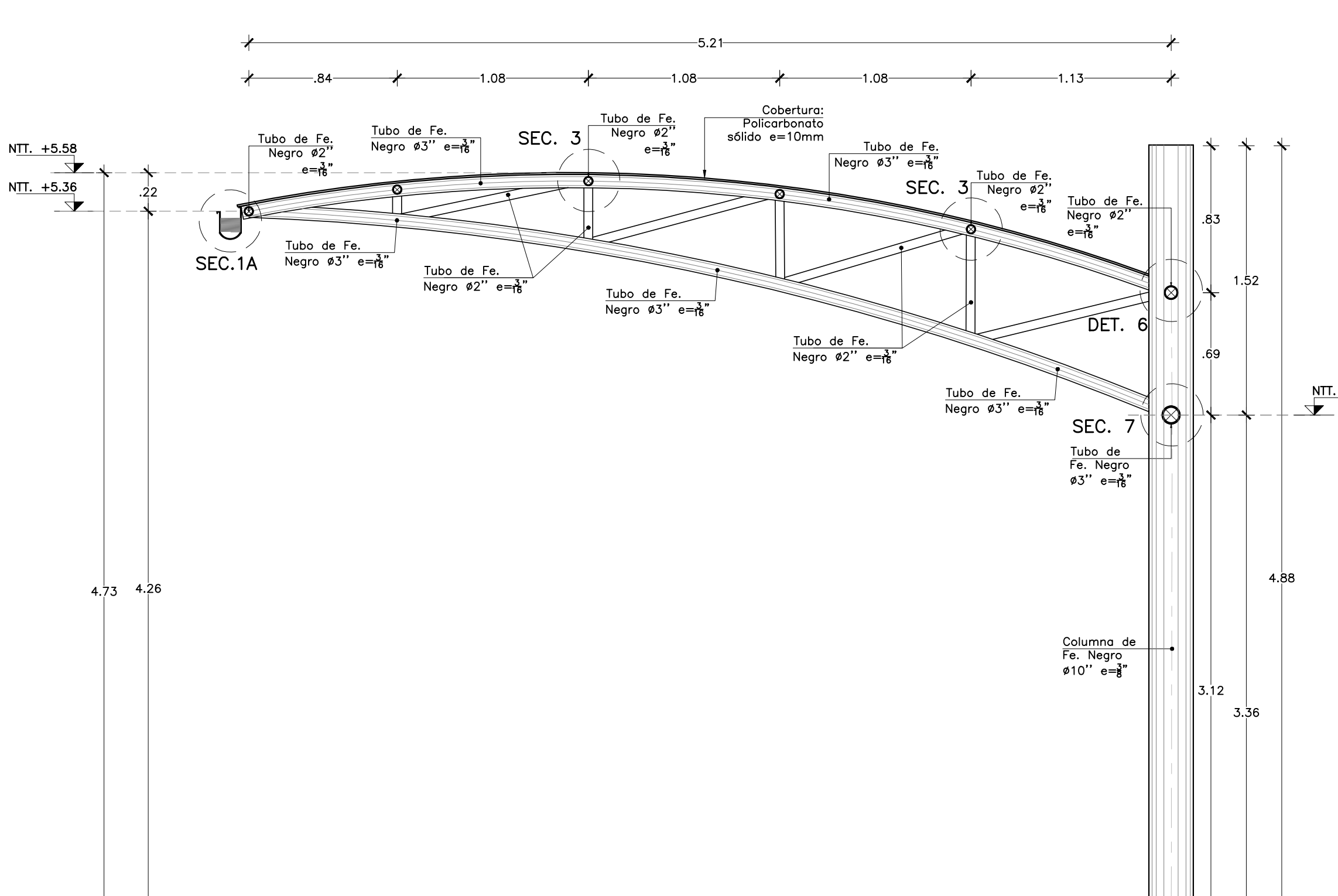
CORTE A-A - COBERTURA N°4 Esc. 1:25
