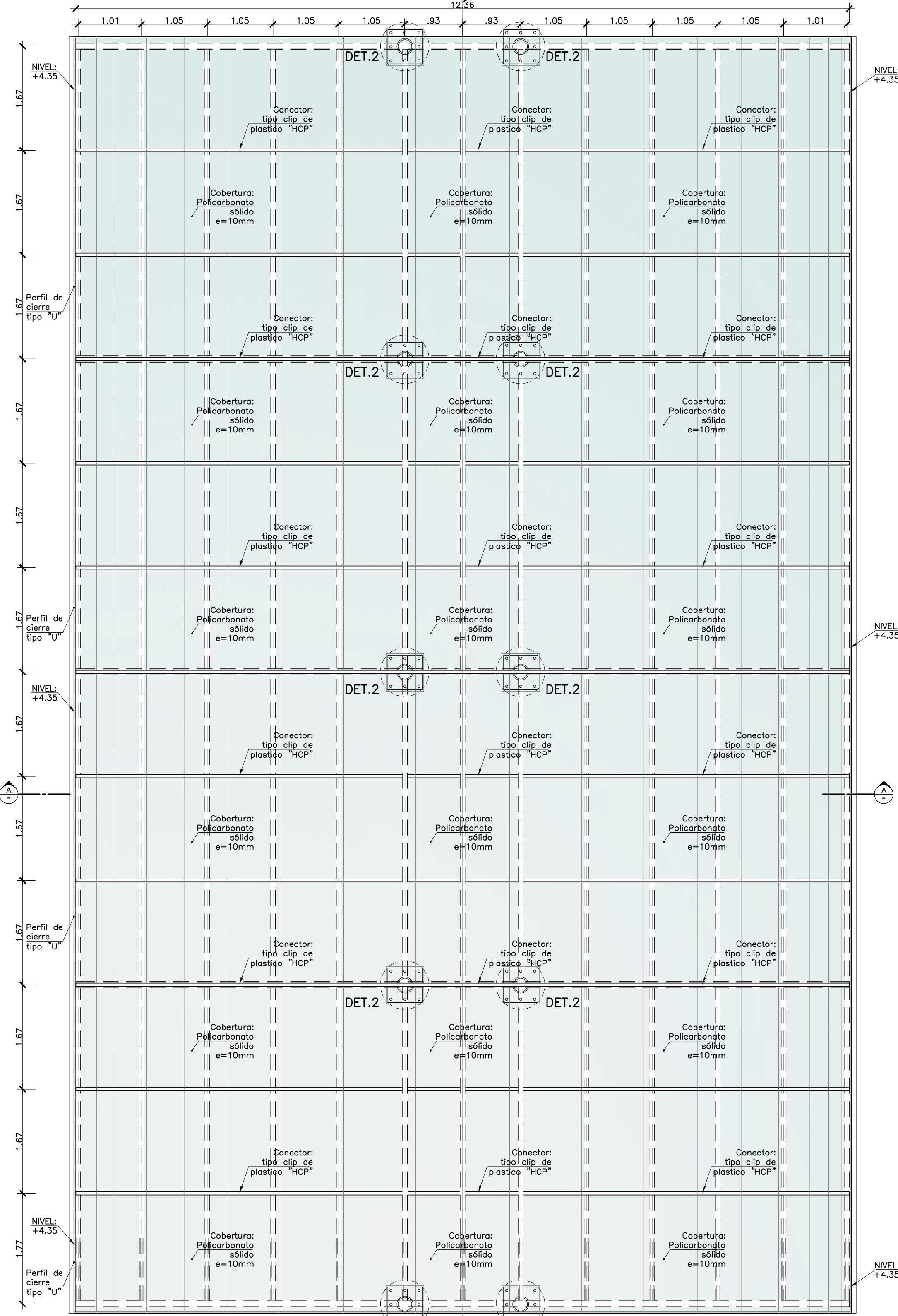
COBERTURA N°3 PLANTA DE COBERTURA Esc. 1:25
