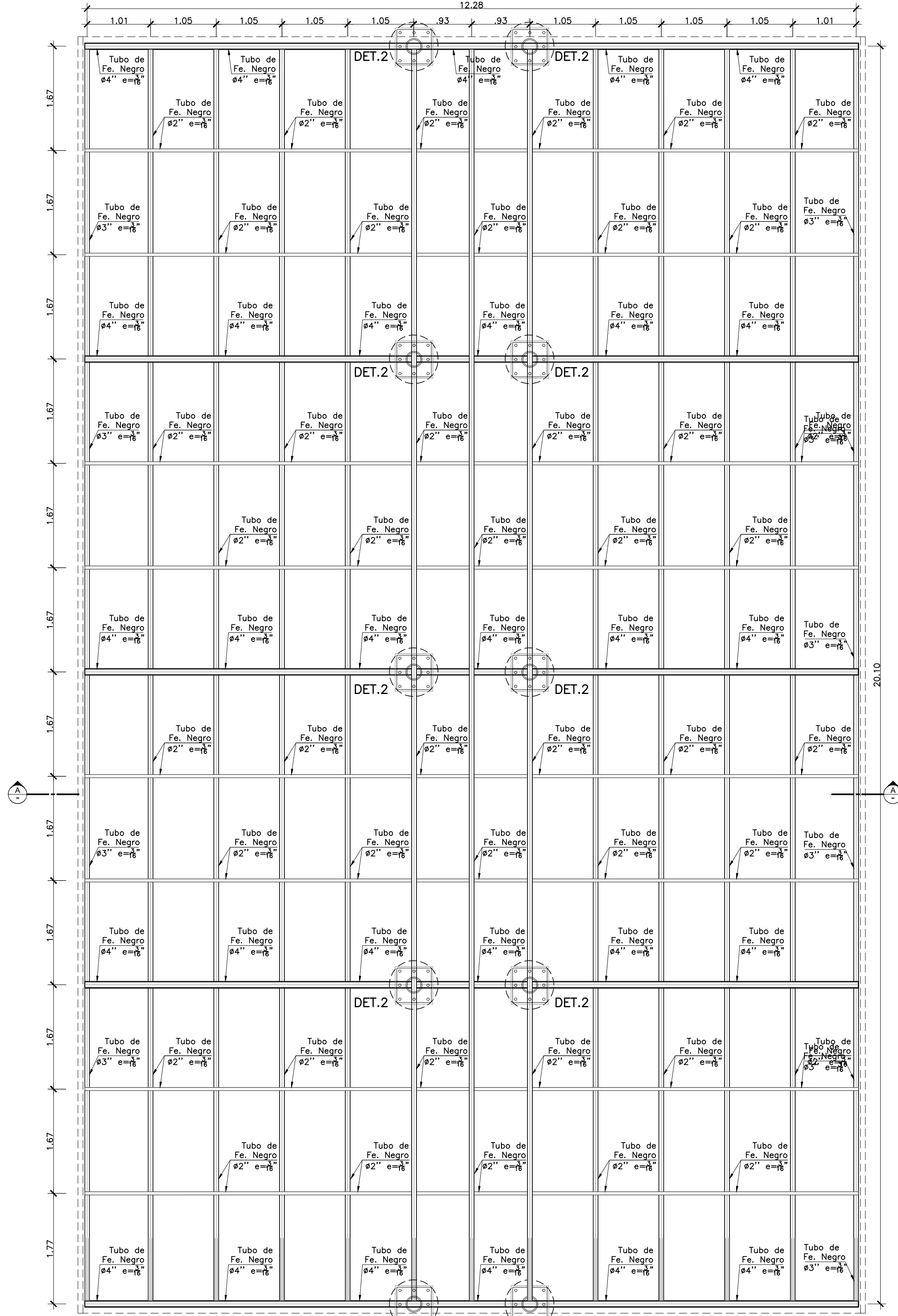
COBERTURA N°3 PLANTA ESTRUCTURAS Esc. 1:25
