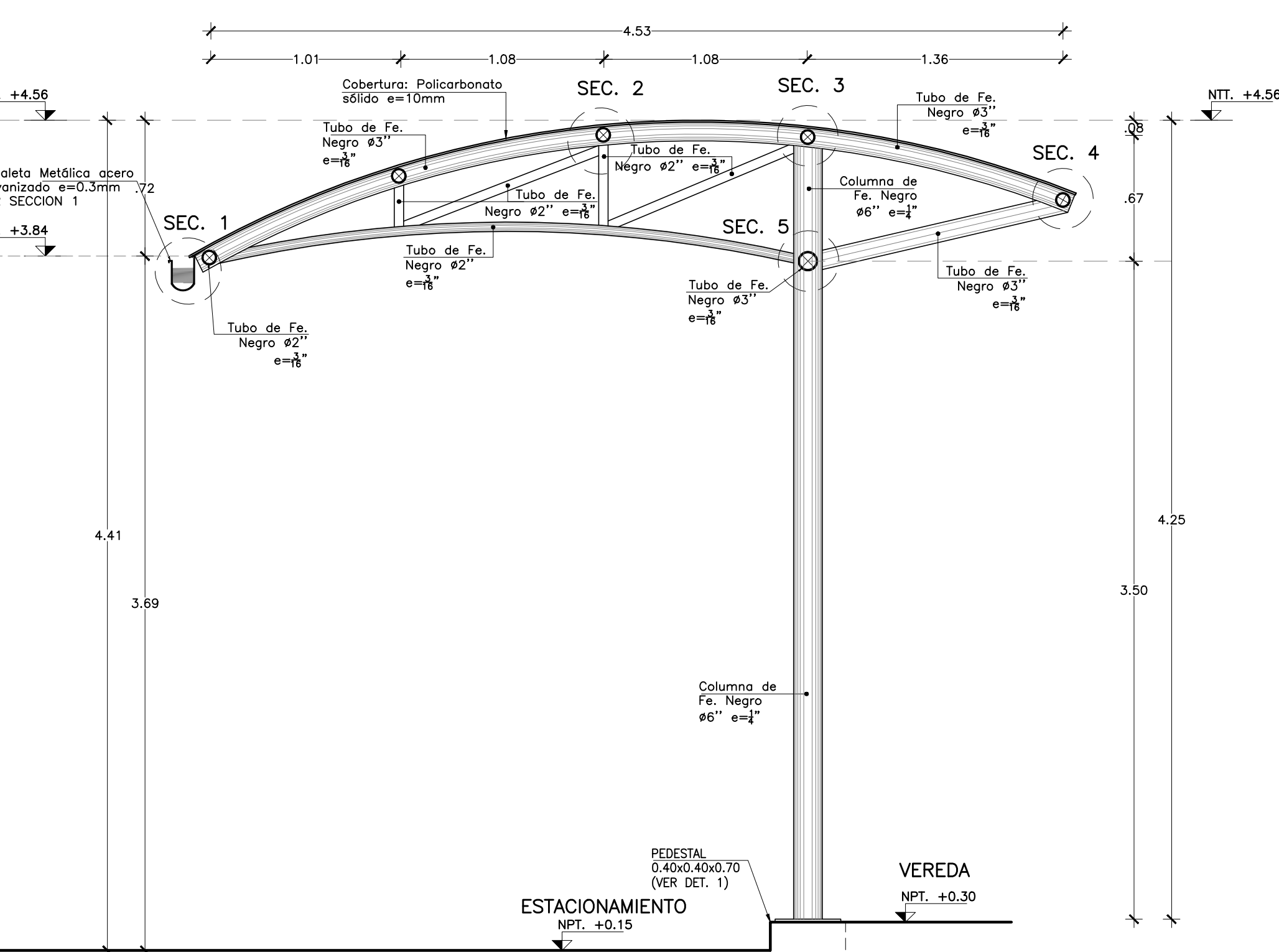
CORTE A-A - COBERTURA N°2 Esc. 1:25
