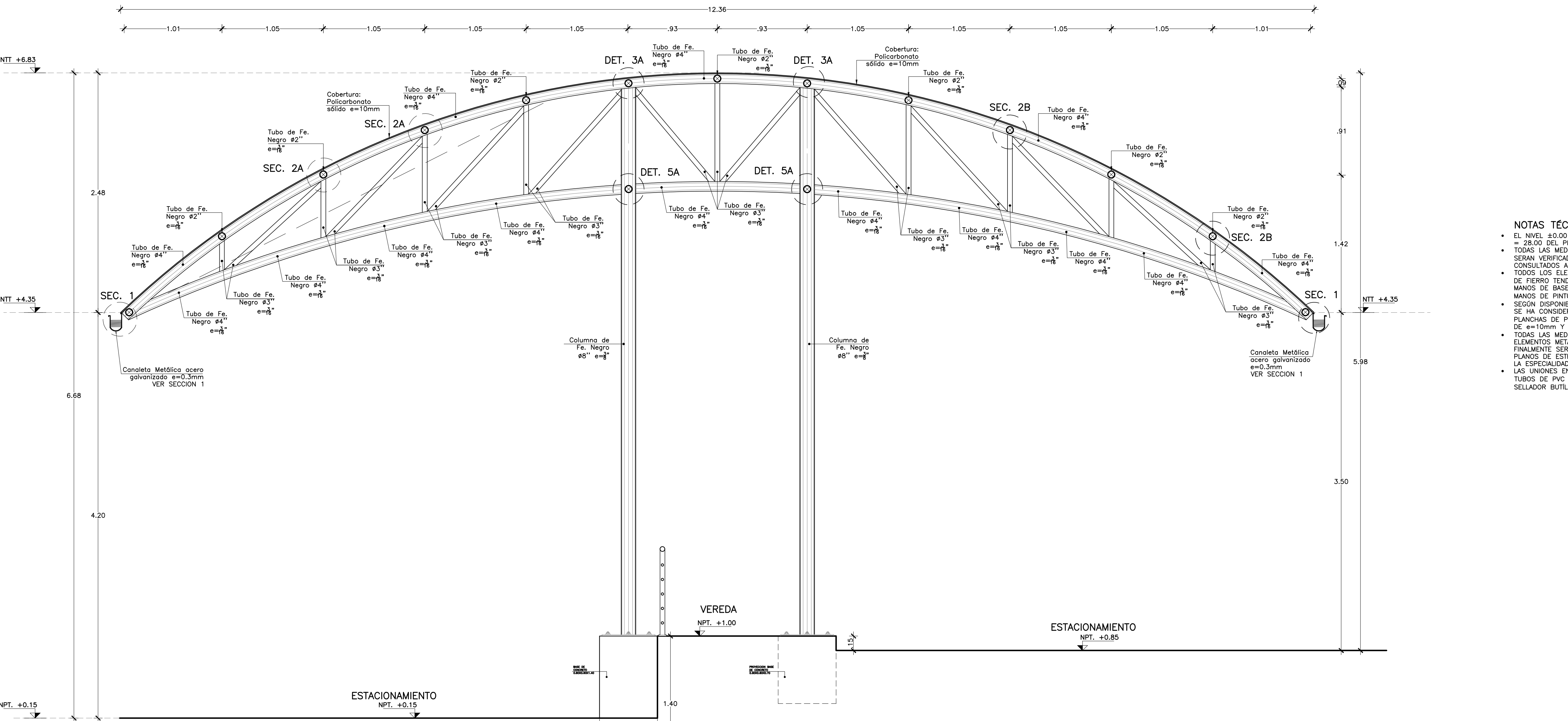
CORTE A-A - COBERTURA N°3 Esc. 1:25
