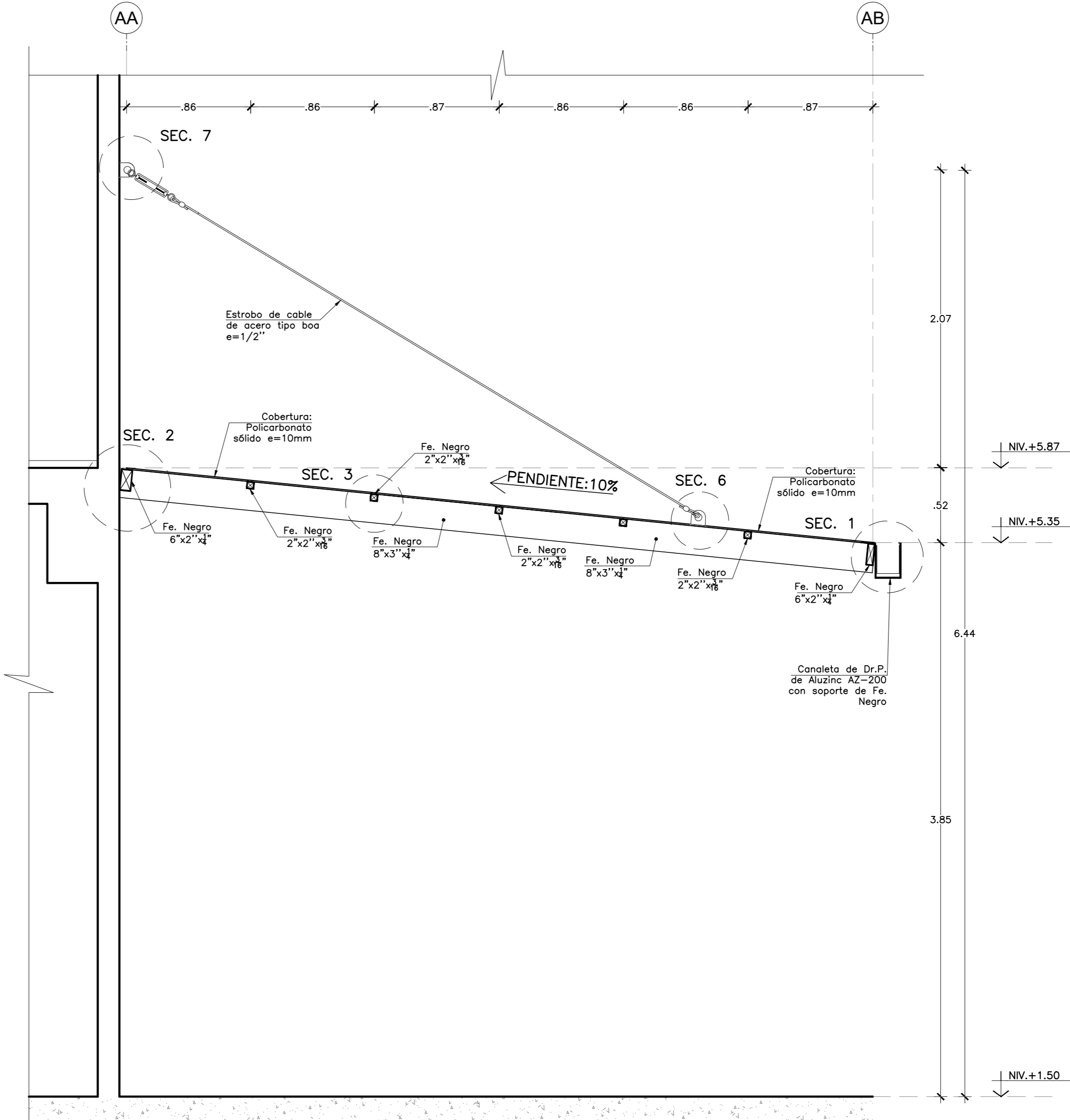
CORTE A-A - MARQUESINA N° 1 Esc. 1:25
