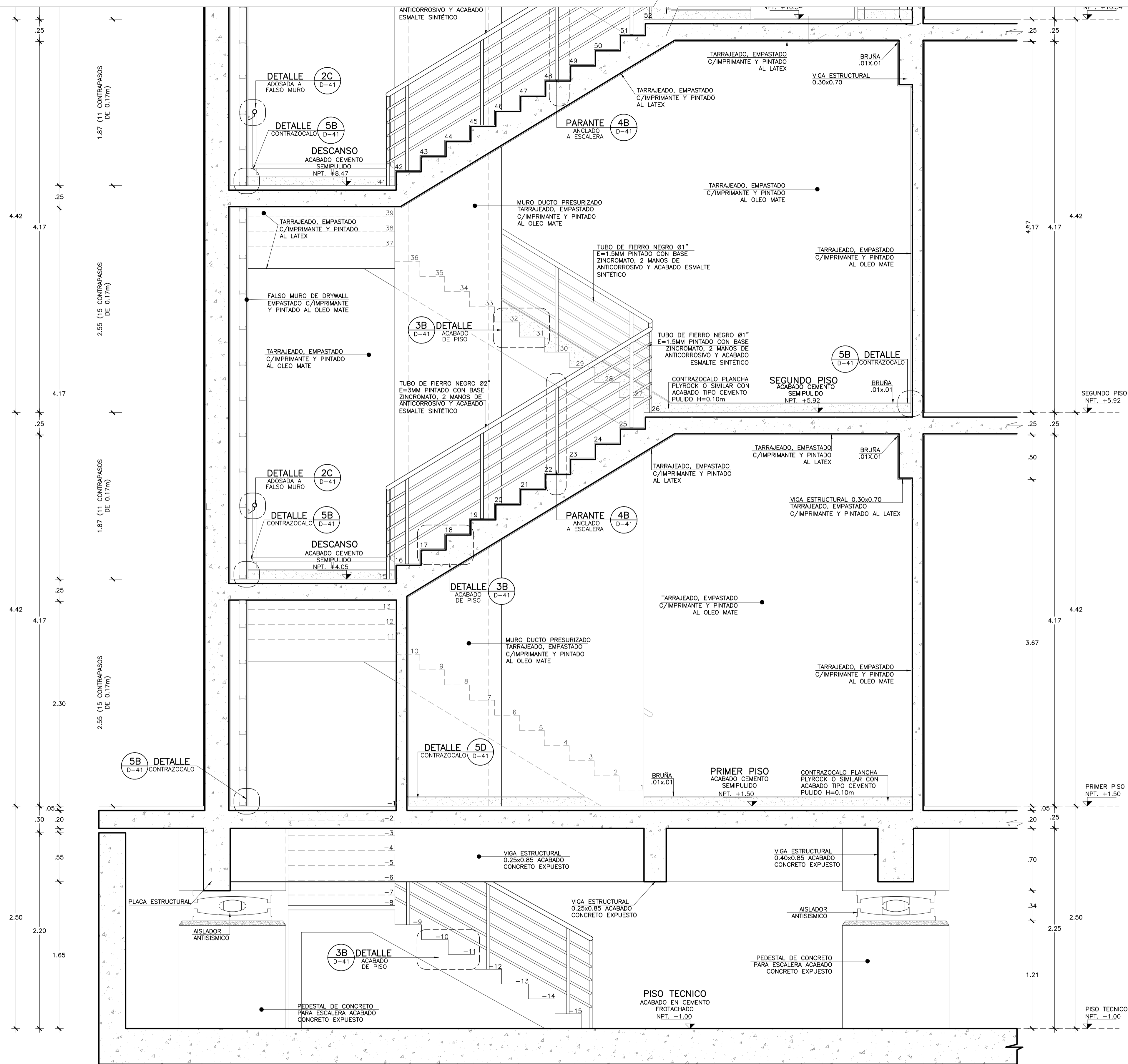
ESCALERA PROTEGIDA N° 2 CORTE 1-1 Esc. 1:25
