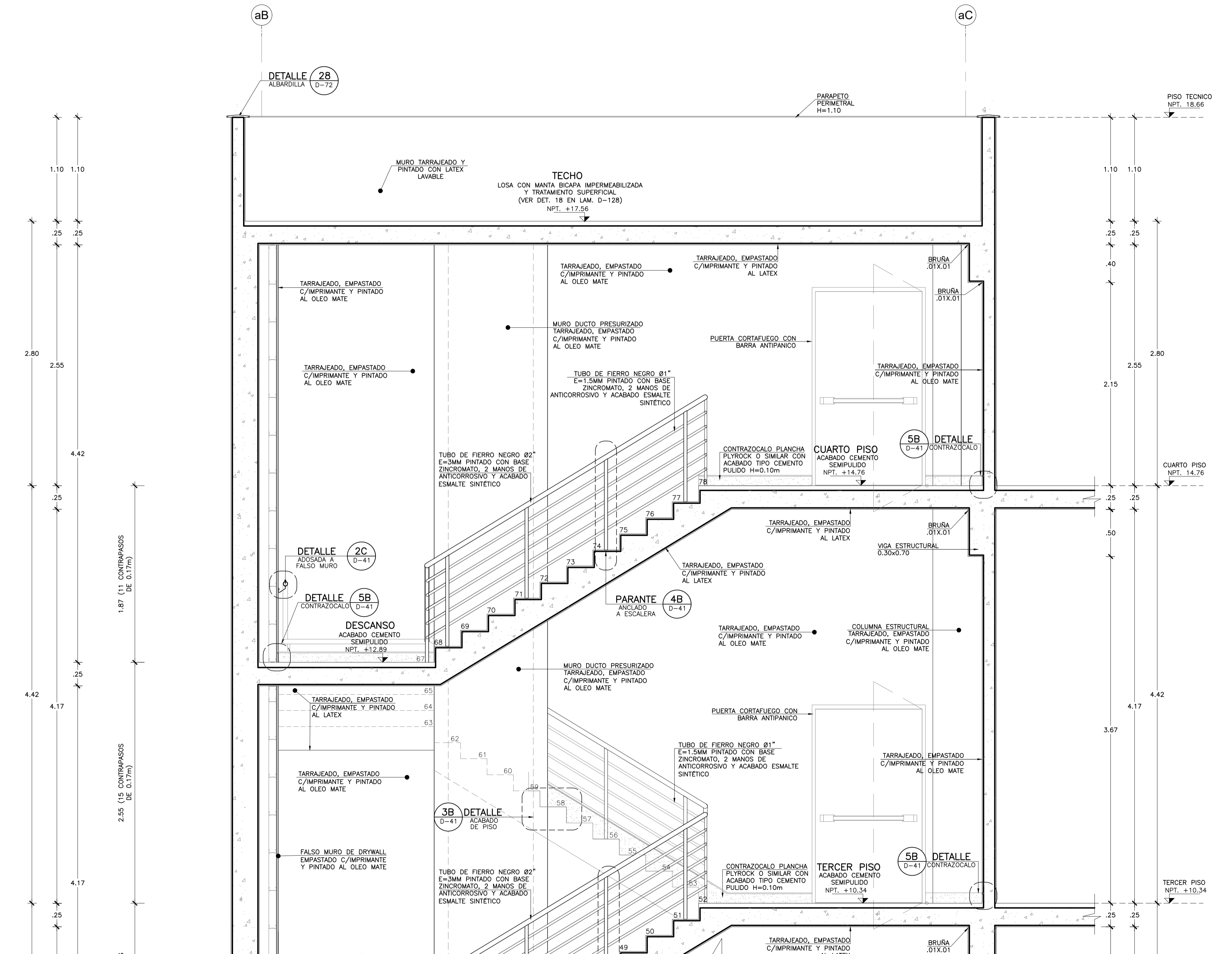
ESCALERA PROTEGIDA N° 02 CORTE 1-1 Esc. 1:25
