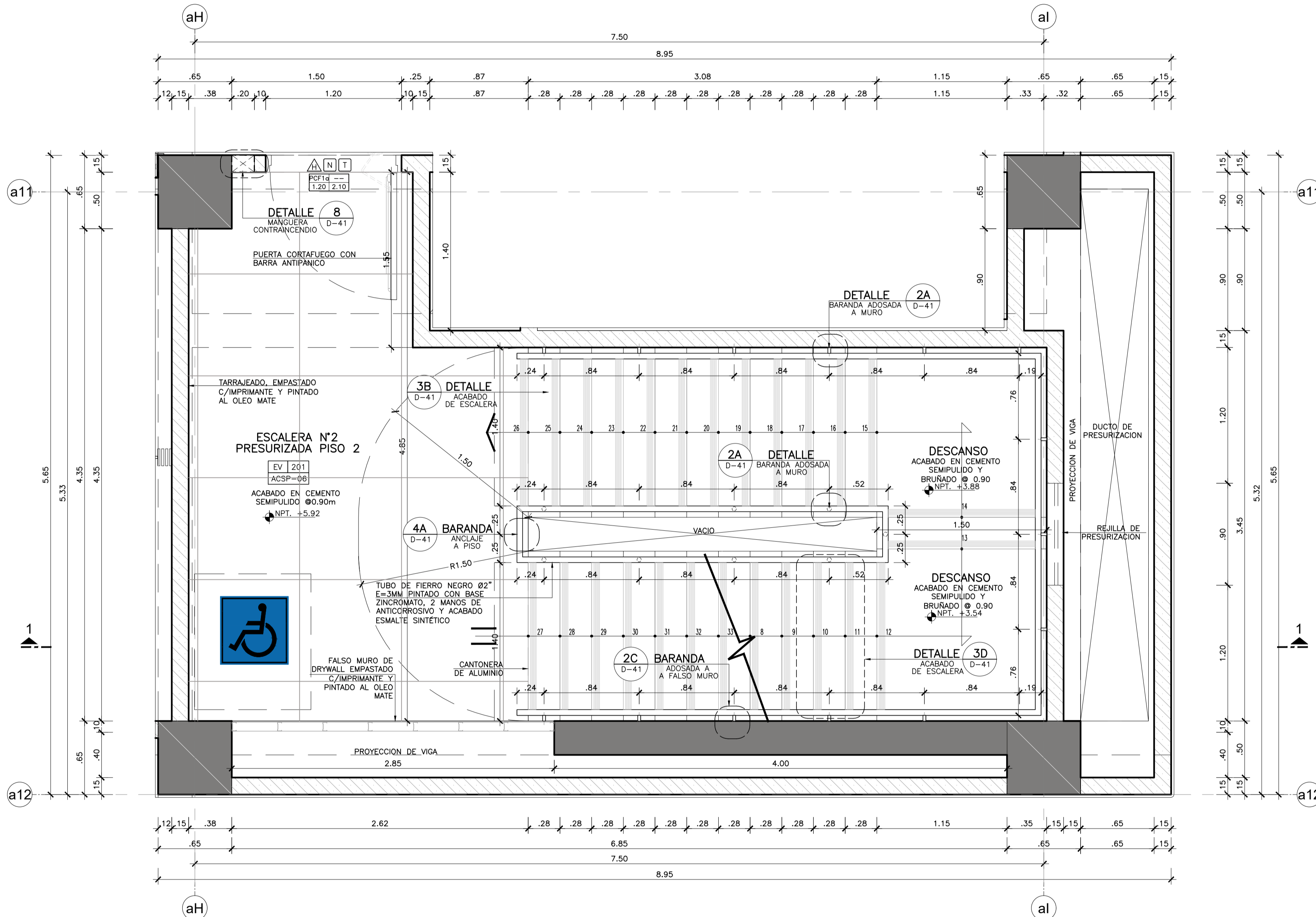
ESCALERA PROTEGIDA N° 03 SEGUNDO PISO (NPT+5.92) Esc. 1:25
