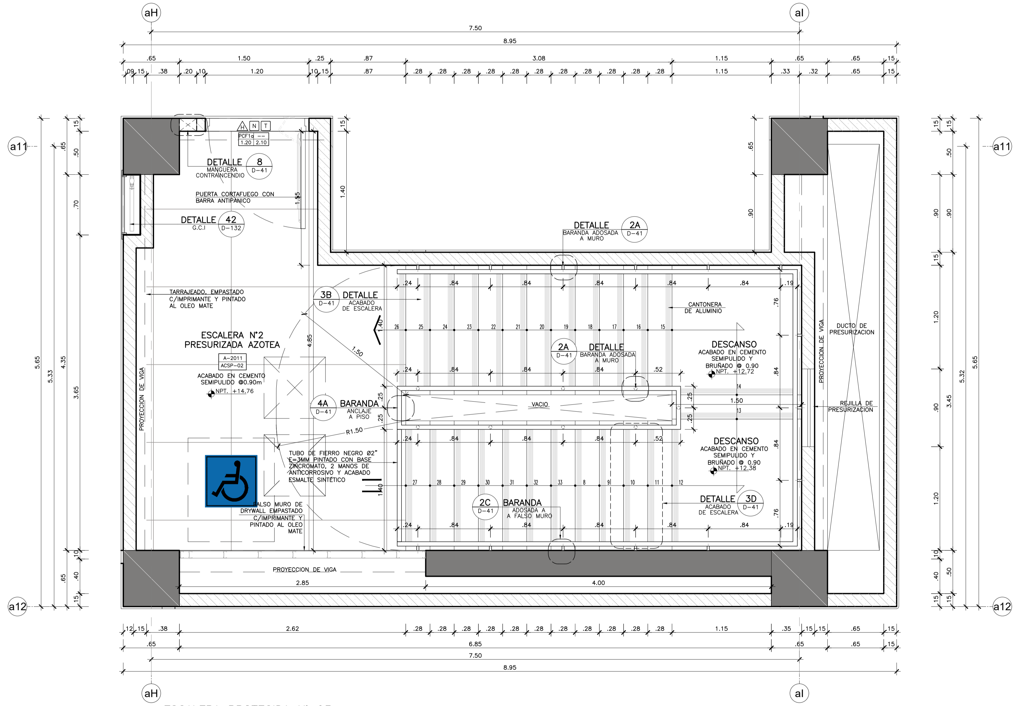
ESCALERA PROTEGIDA N° 03 PISO AZOTEA (NPT+14.76) Esc. 1:25
