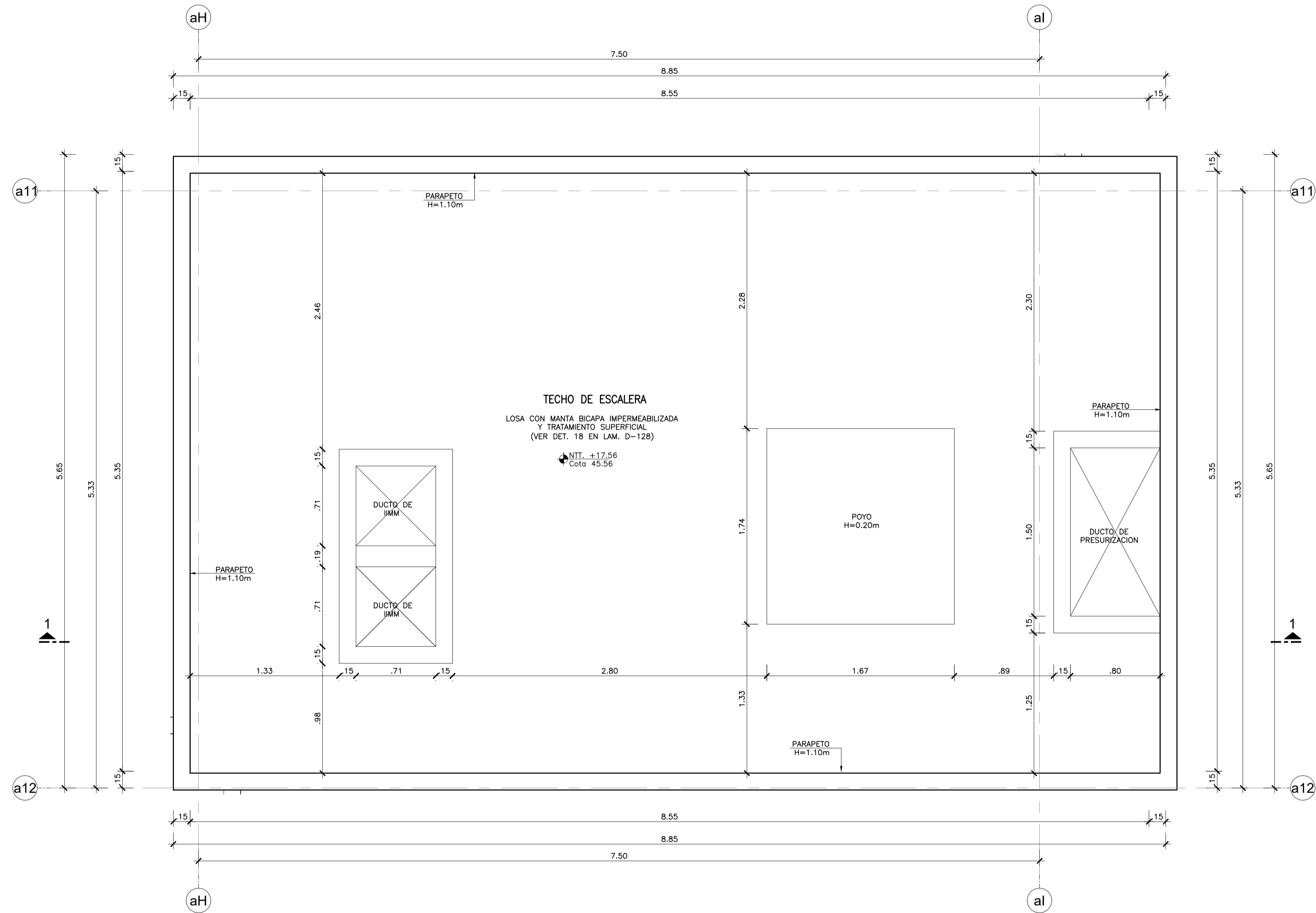
ESCALERA PROTEGIDA N° 03 TECHO (NPT+19.18) Esc. 1:25
