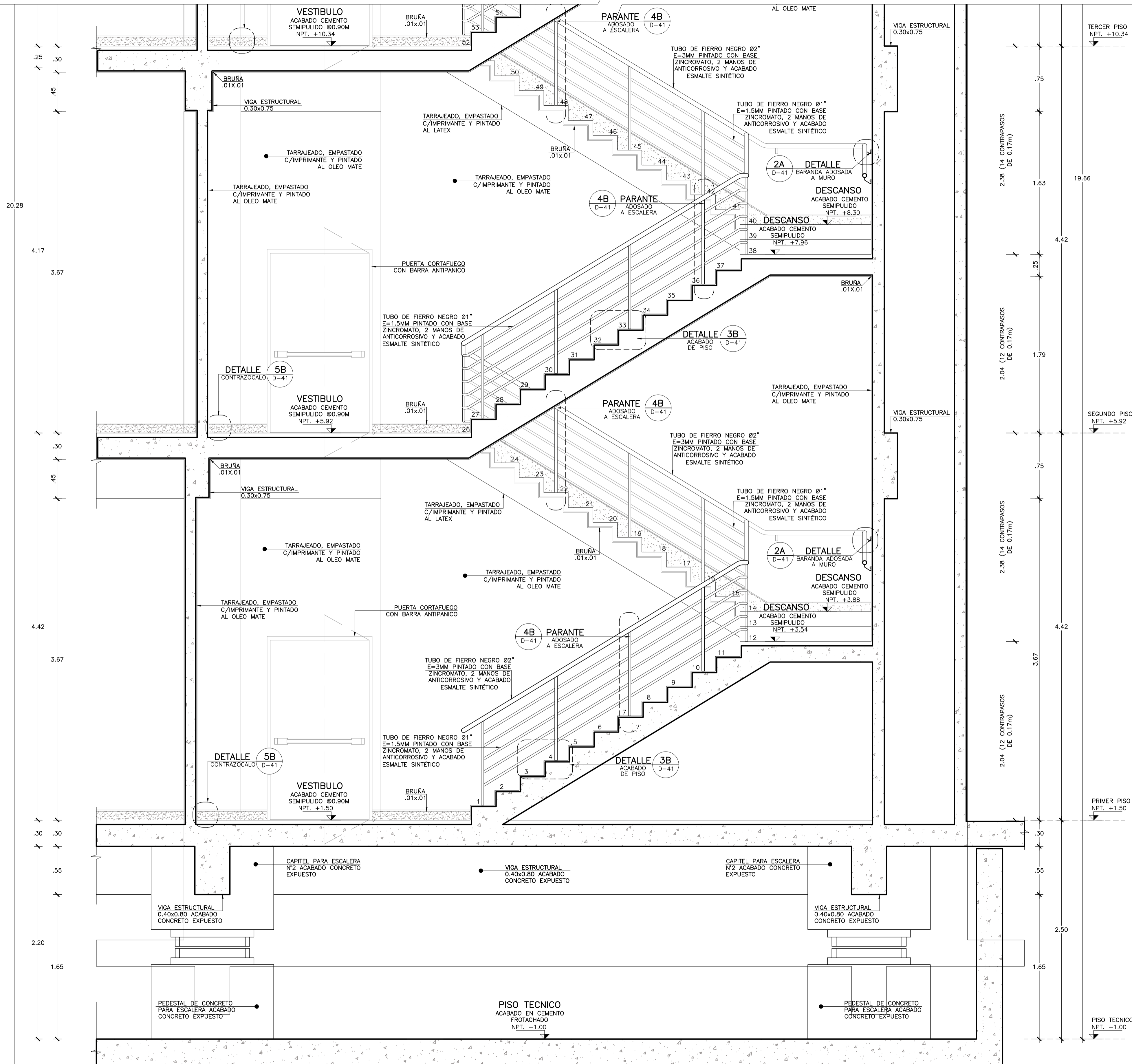
ESCALERA PROTEGIDA N° 03 CORTE 1-1 Esc. 1:25
