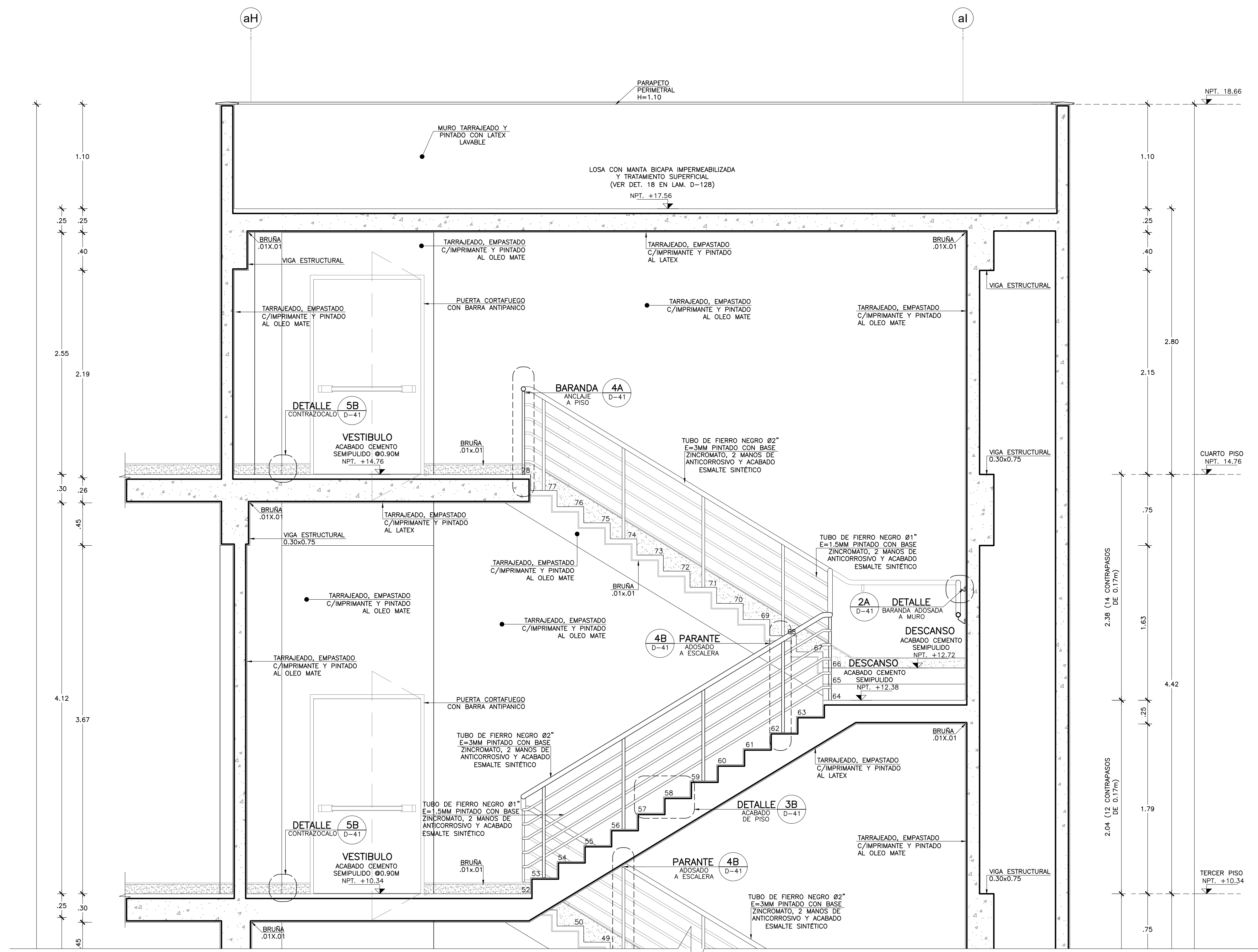
ESCALERA PROTEGIDA N° 03 CORTE 1-1 Esc. 1:25
