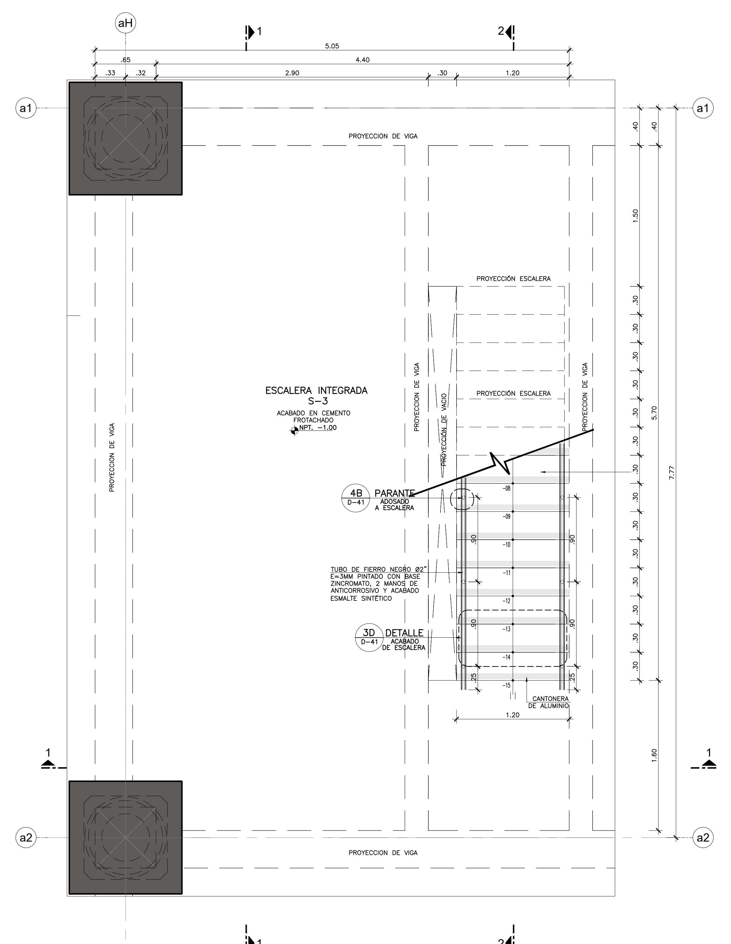
ESCALERA PROTEGIDA N° 04 PISO TECNICO (NPT-1.00) Esc. 1:25
