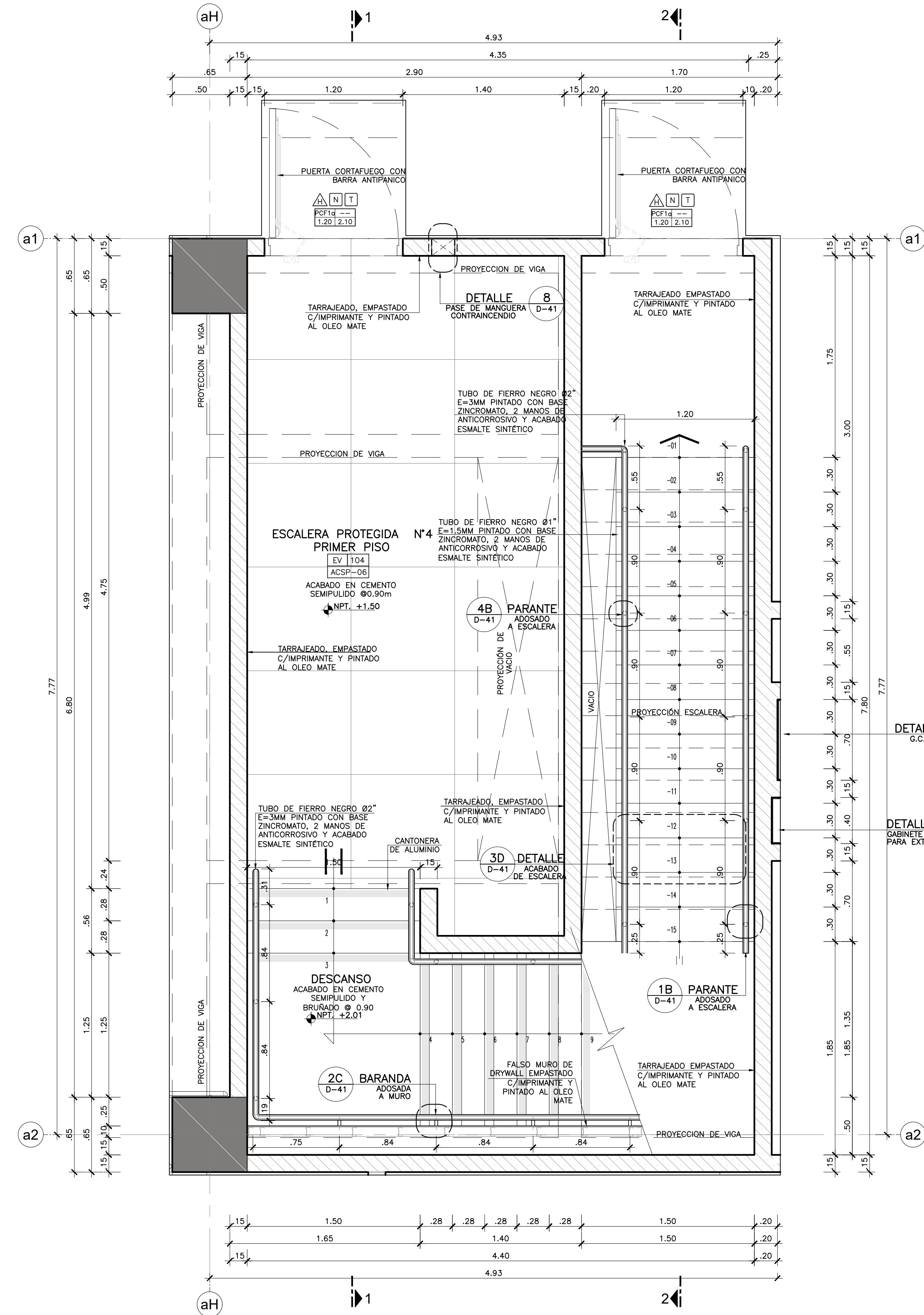
ESCALERA PROTEGIDA N° 04 PISO PRIMER PISO (NPT+1.50) Esc. 1:25
