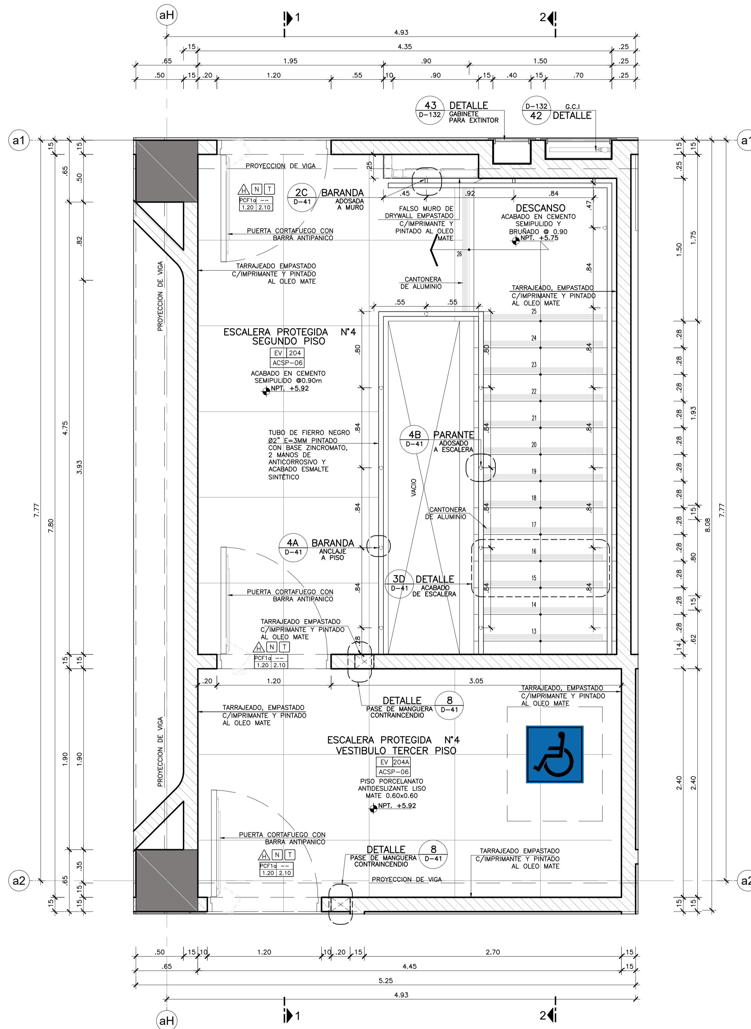
ESCALERA PROTEGIDA N° 04 SEGUNDO PISO (NPT+5.92) Esc. 1:25
