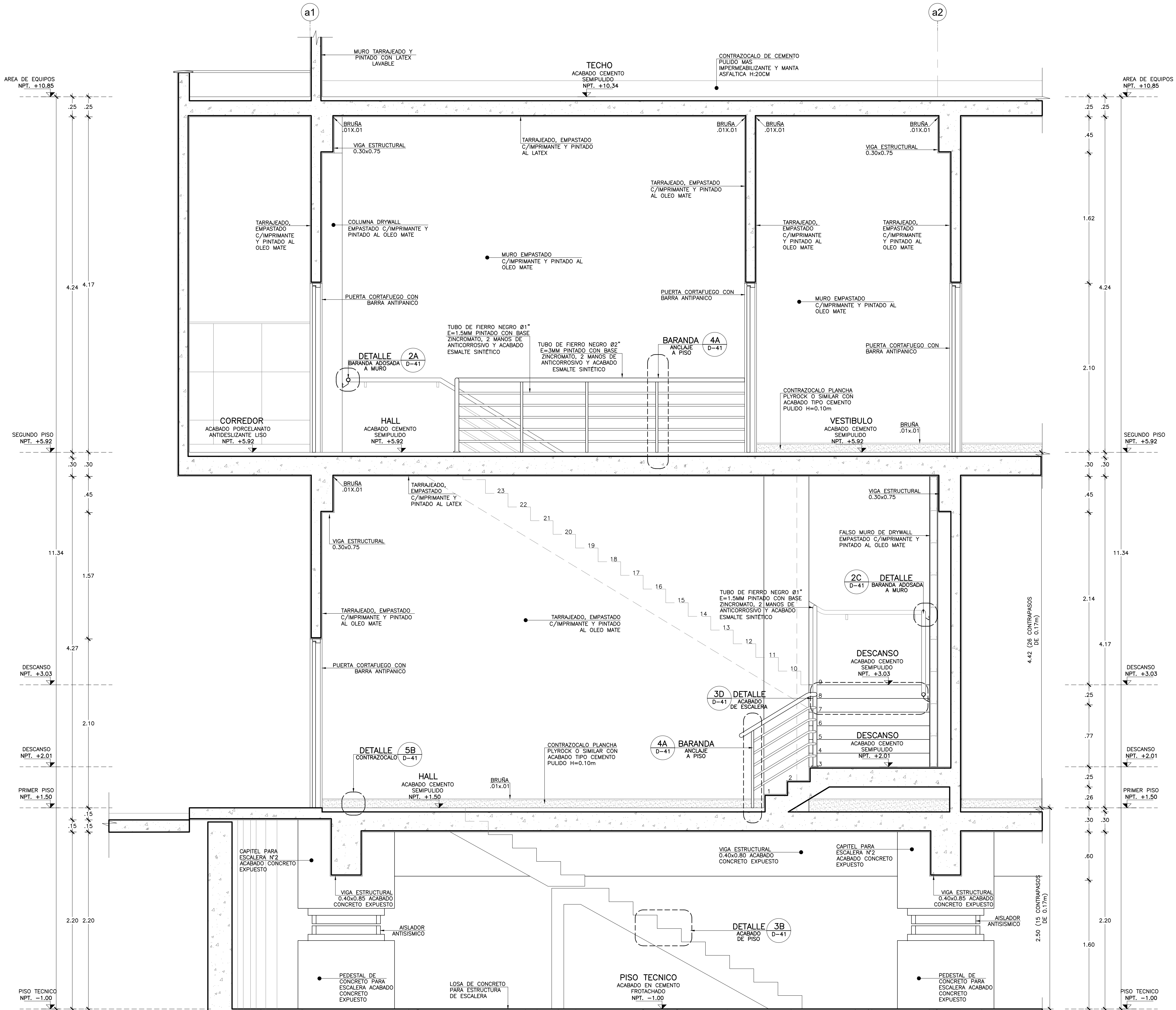
ESCALERA PROTEGIDA N° 4 CORTE 1-1 Esc. 1:25
