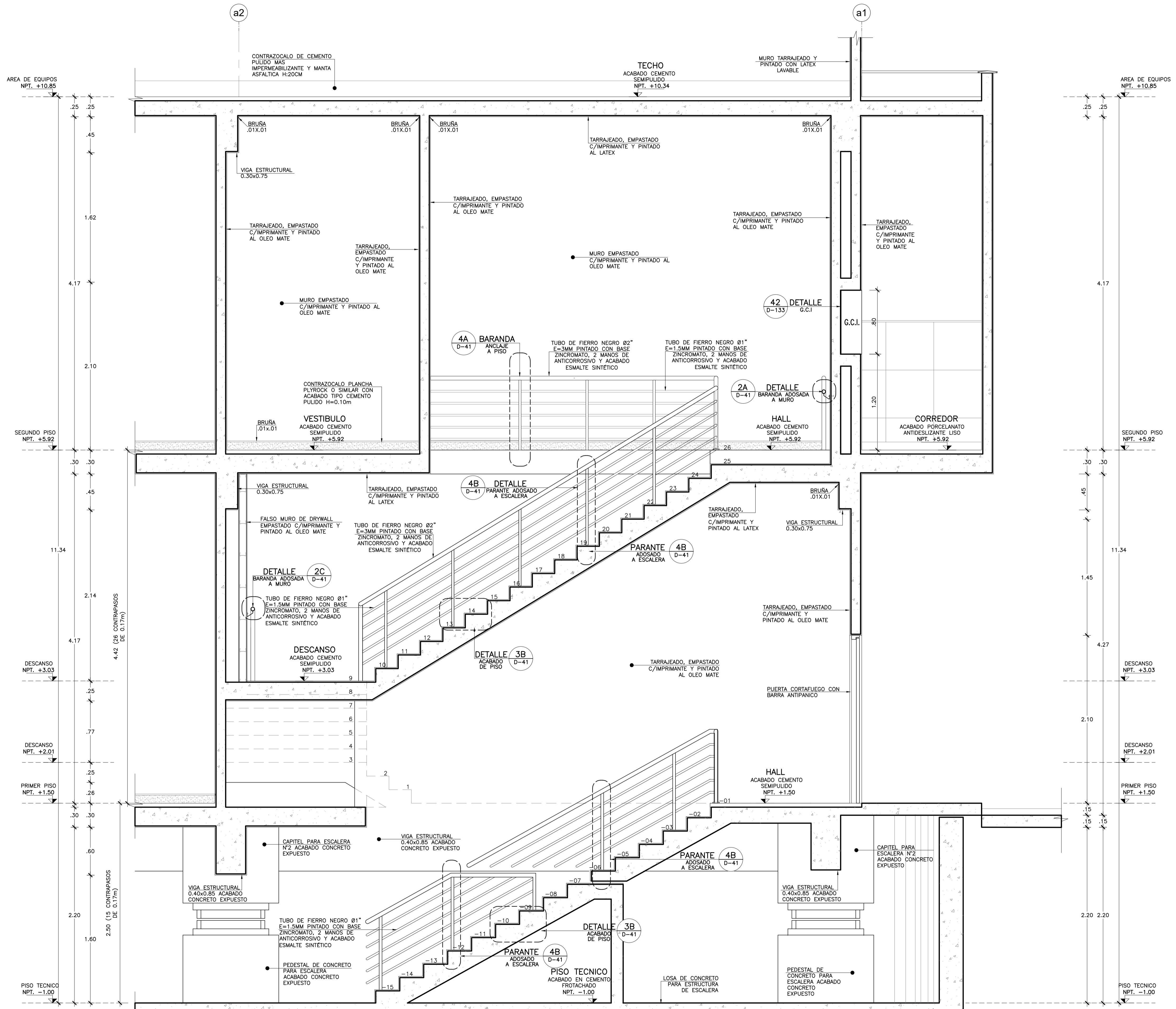
ESCALERA PROTEGIDA N° 4 CORTE 2-2 Esc. 1:25
