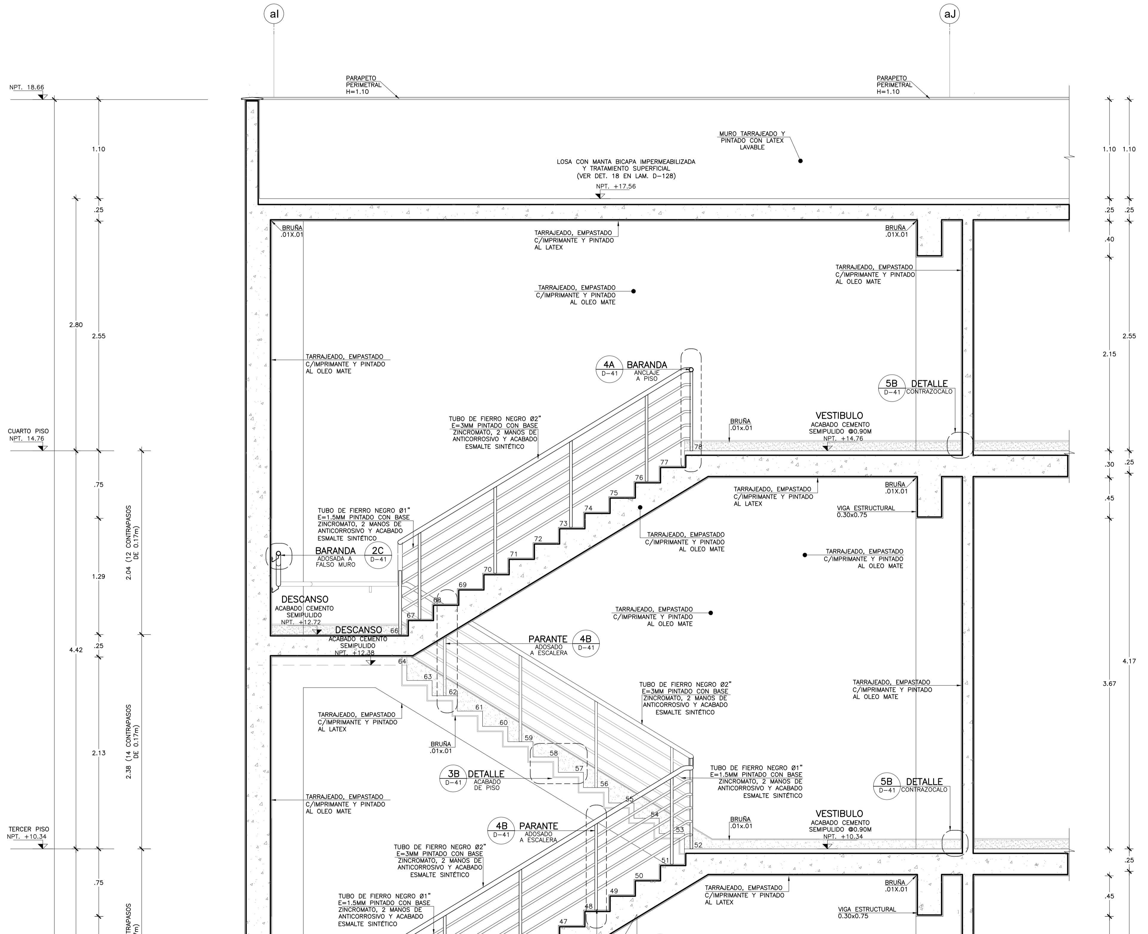
ESCALERA PROTEGIDA N° 05 CORTE 1-1 Esc. 1:25
