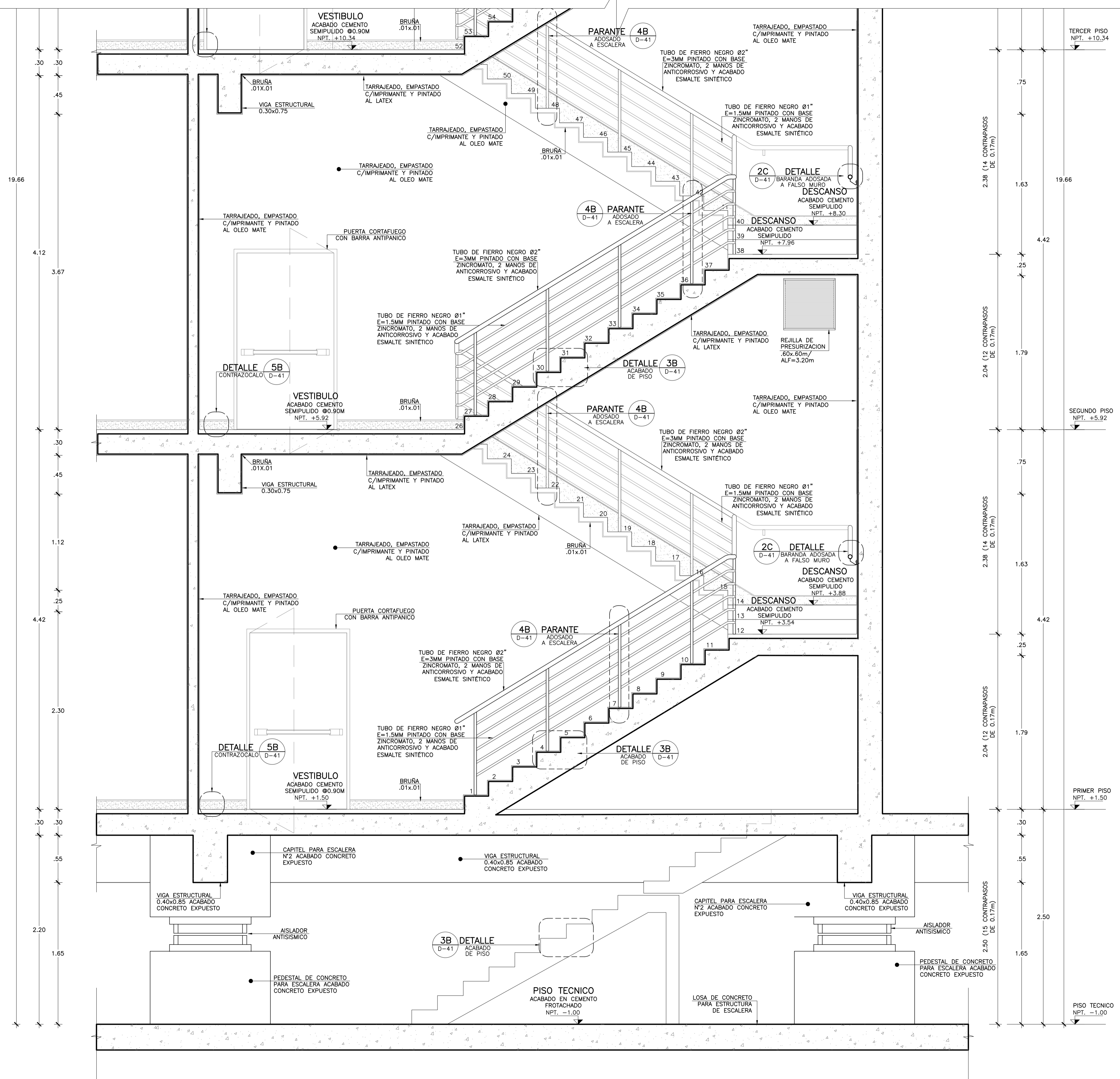
ESCALERA PROTEGIDA N° 05 CORTE 2-2 Esc. 1:25
