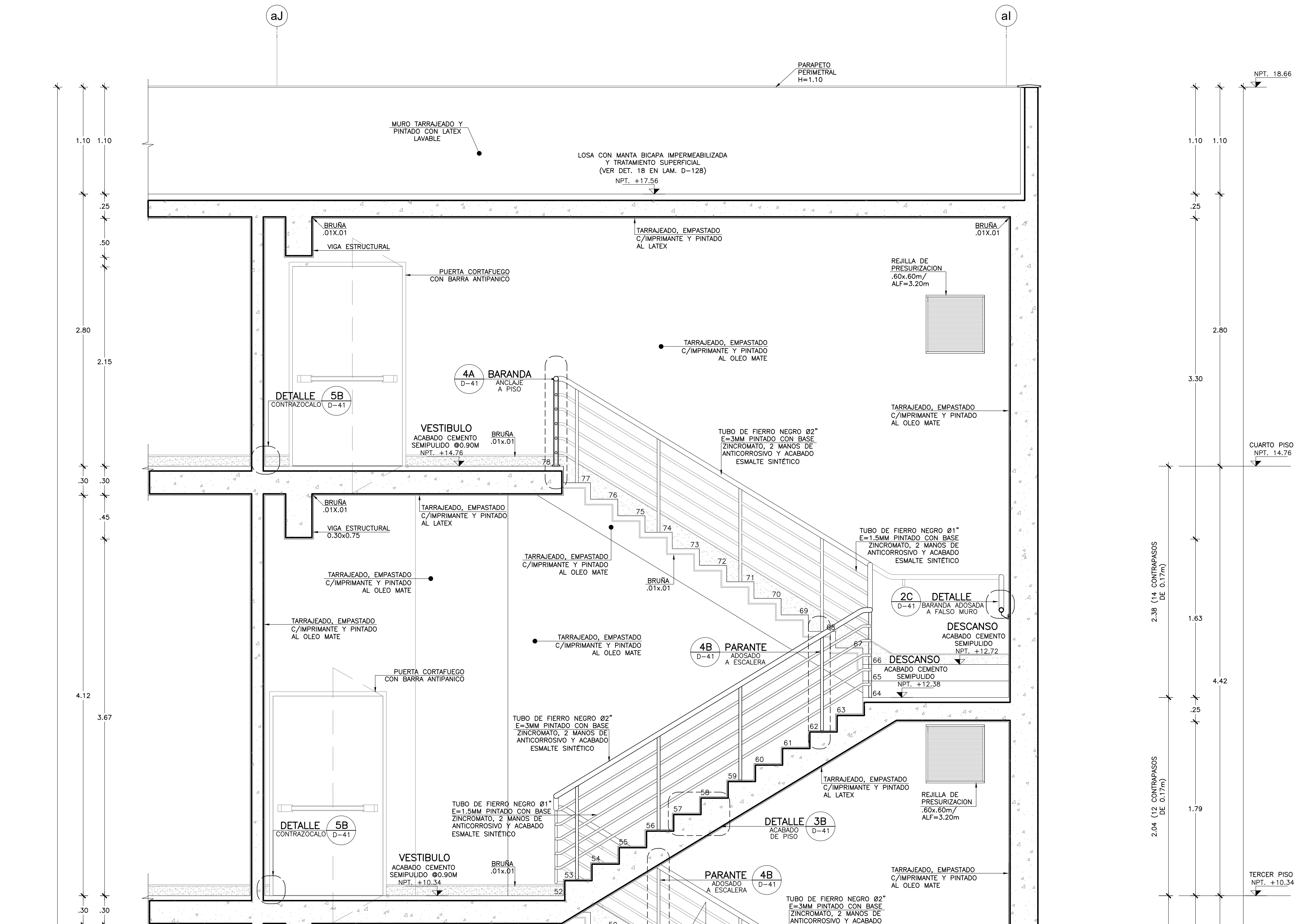
ESCALERA PROTEGIDA N° 05 CORTE 2-2 Esc. 1:25
