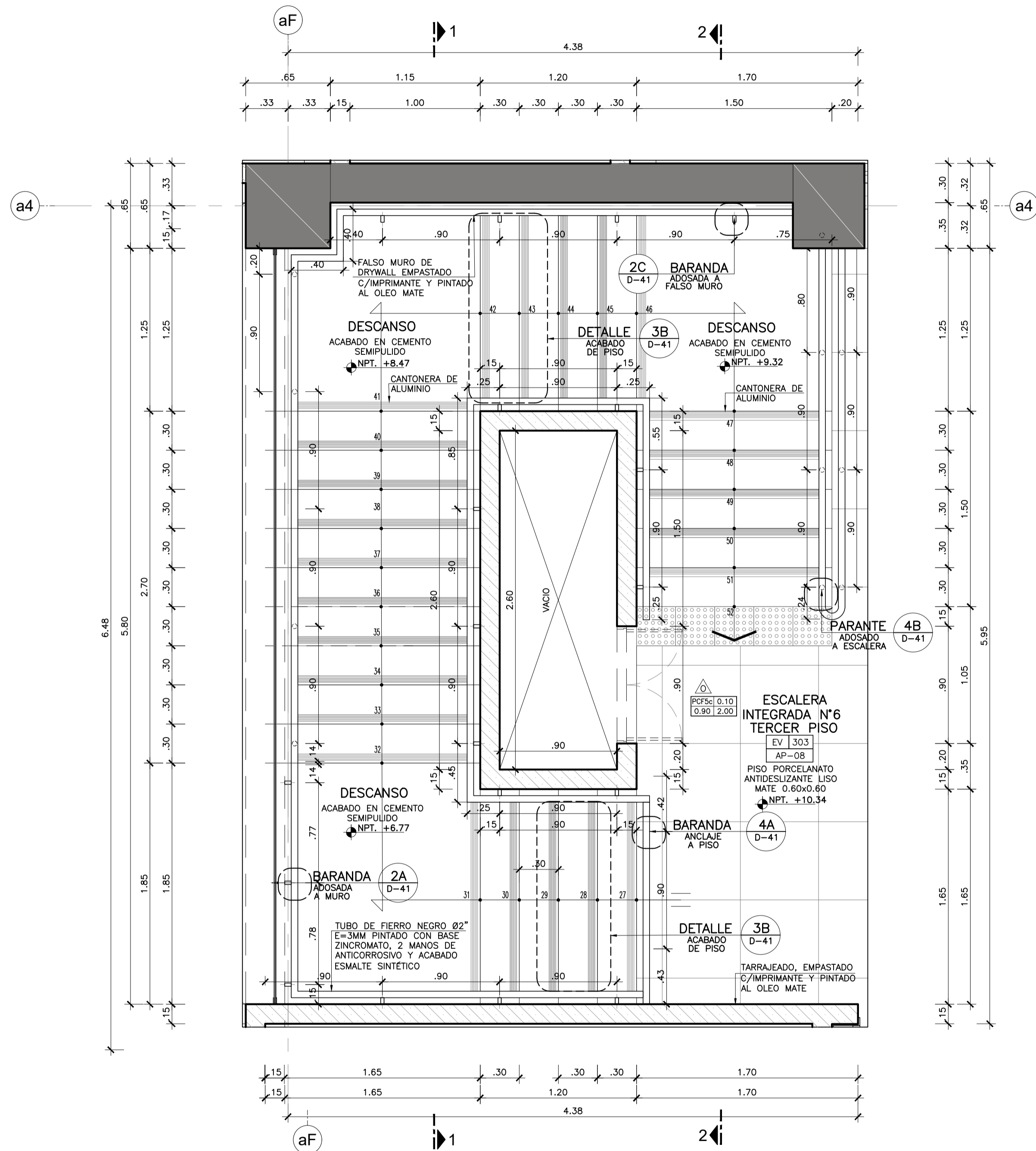
ESCALERA INTEGRADA N° 06 TERCER PISO (NPT+10.34) Esc. 1:25
