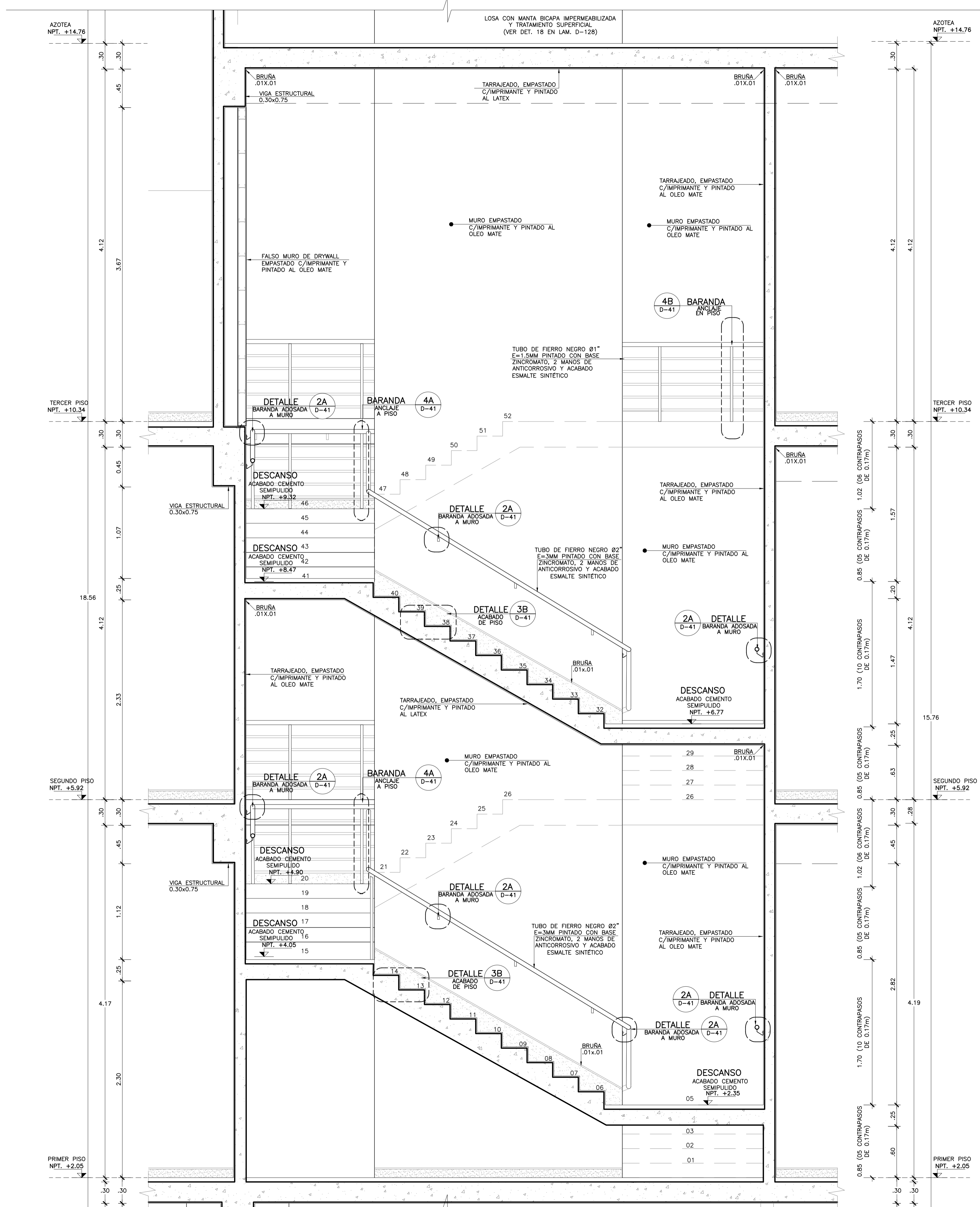
ESCALERA INTEGRADA N° 6 CORTE 1-1 Esc. 1:25
