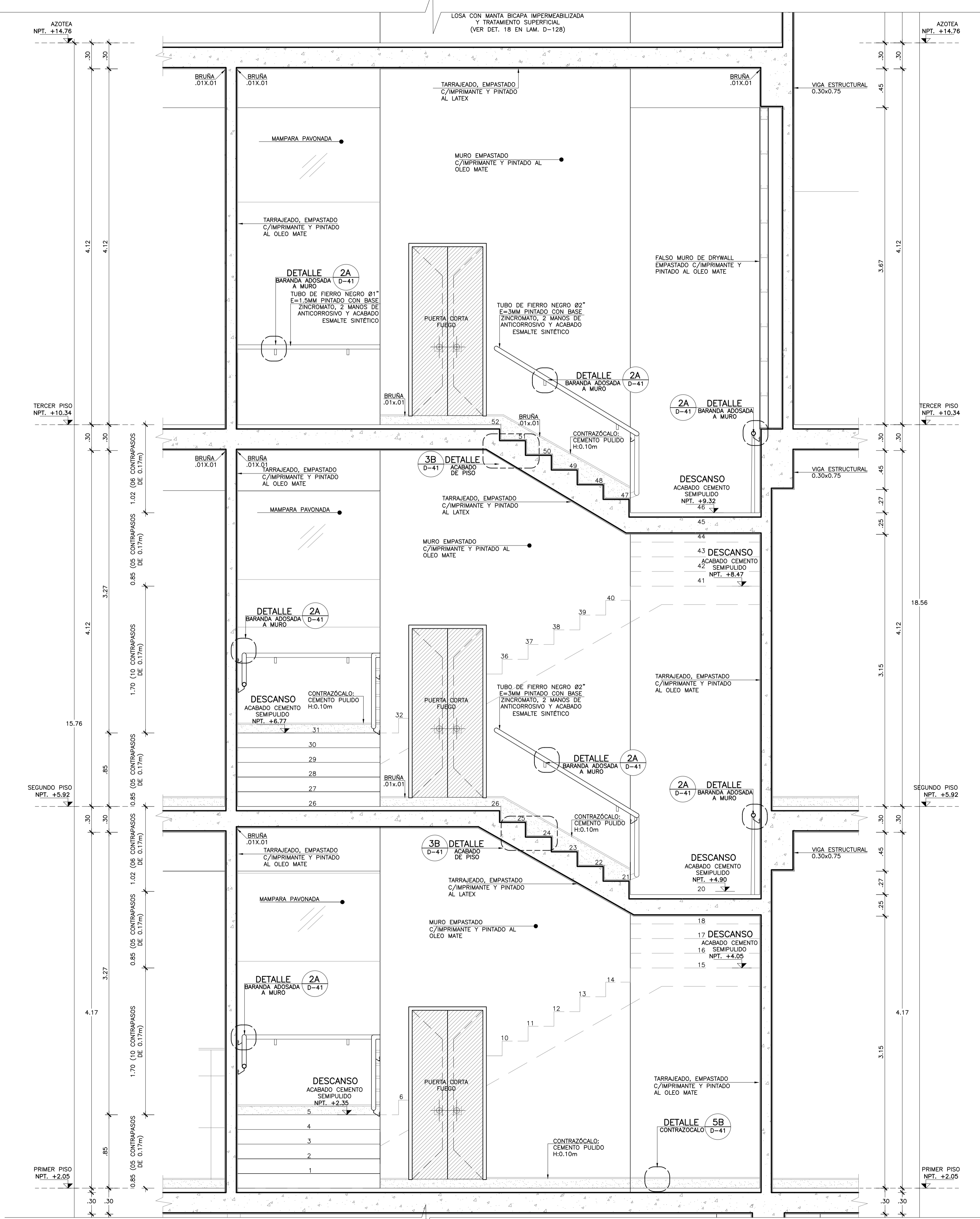
ESCALERA INTEGRADA N° 6 CORTE 2-2 Esc. 1:25
