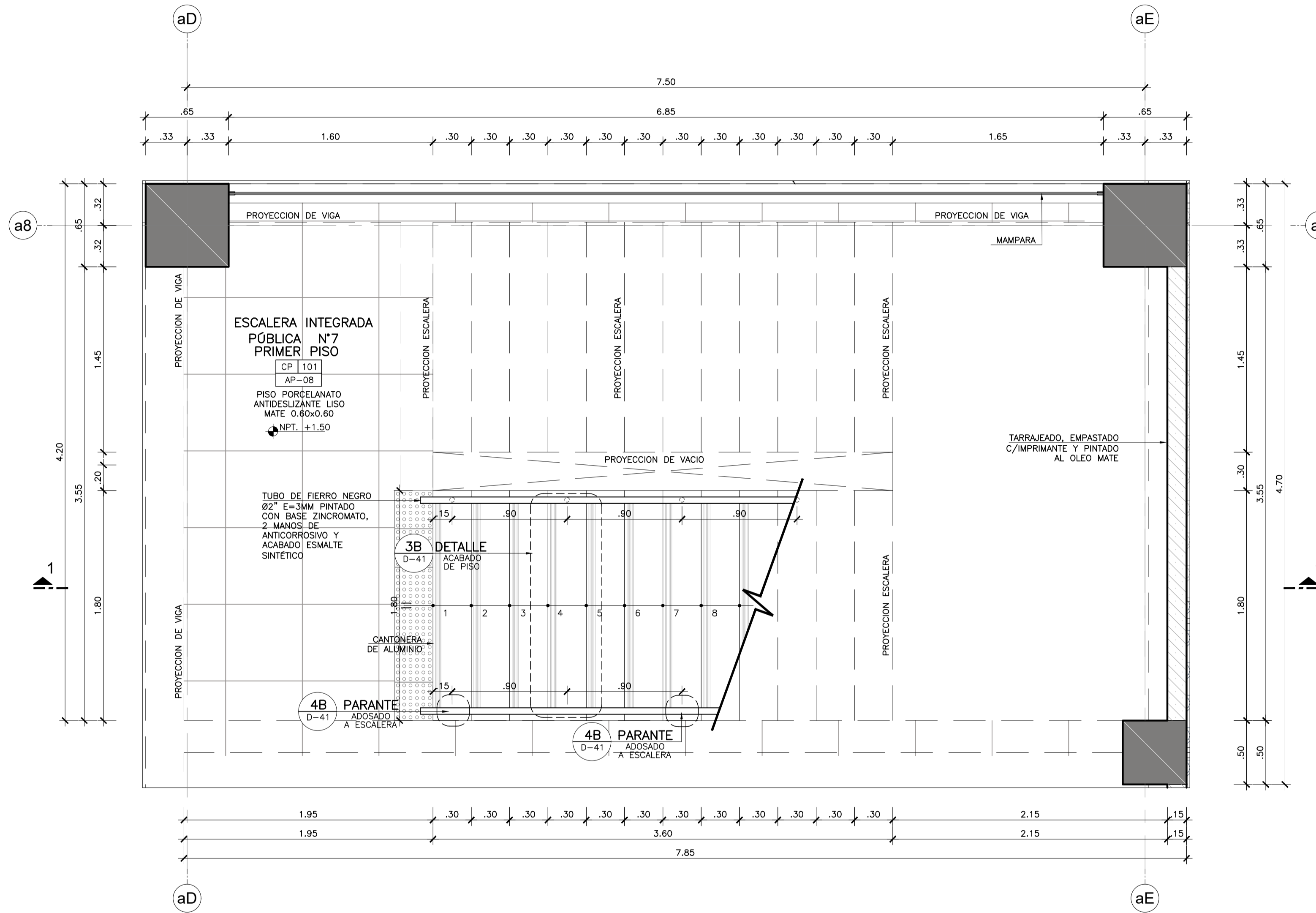
ESCALERA INTEGRADA N° 07 PRIMER PISO (NPT+1.50) Esc. 1:25
