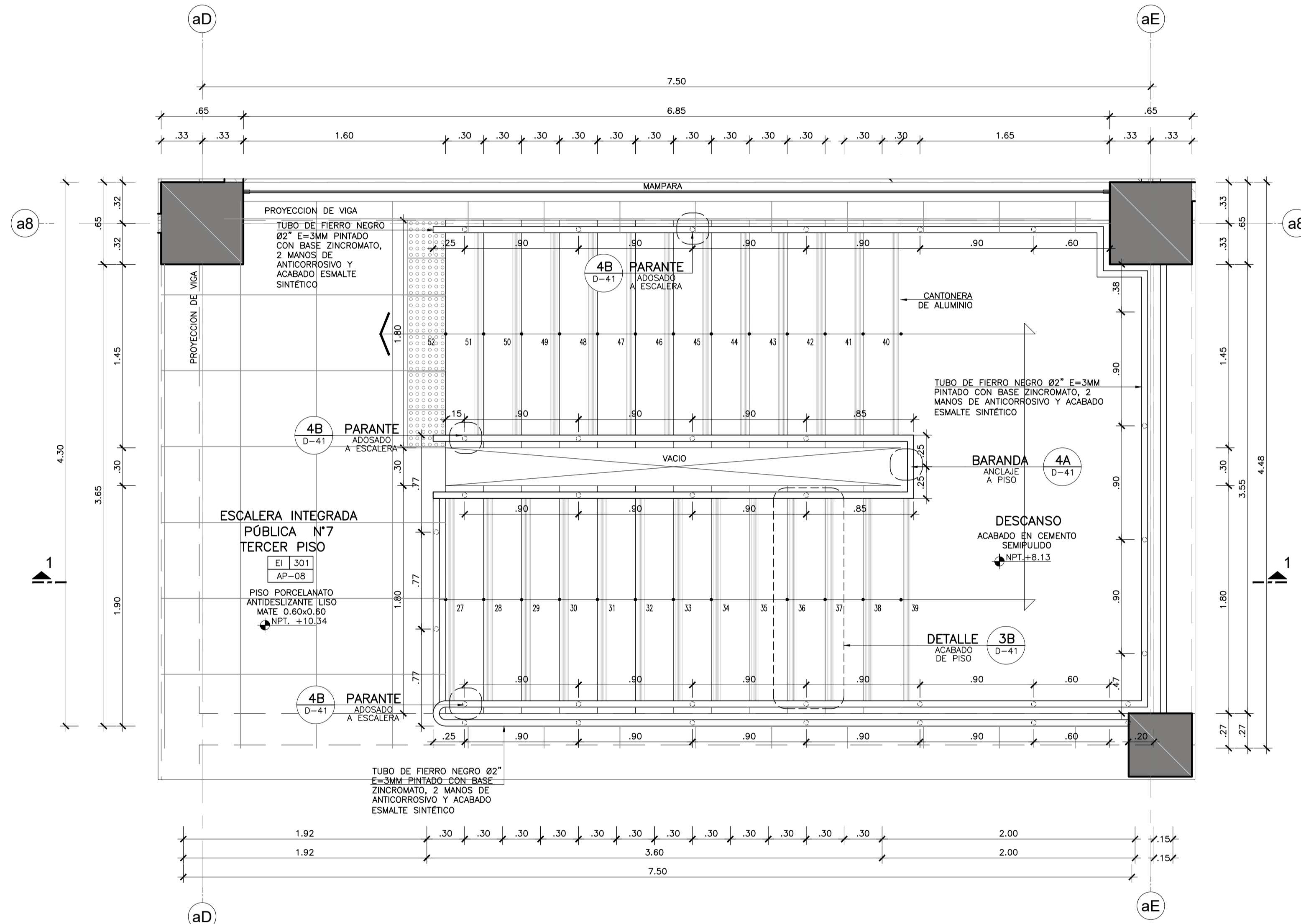
ESCALERA INTEGRADA N° 07 TERCER PISO (NPT+10.34) Esc. 1:25
