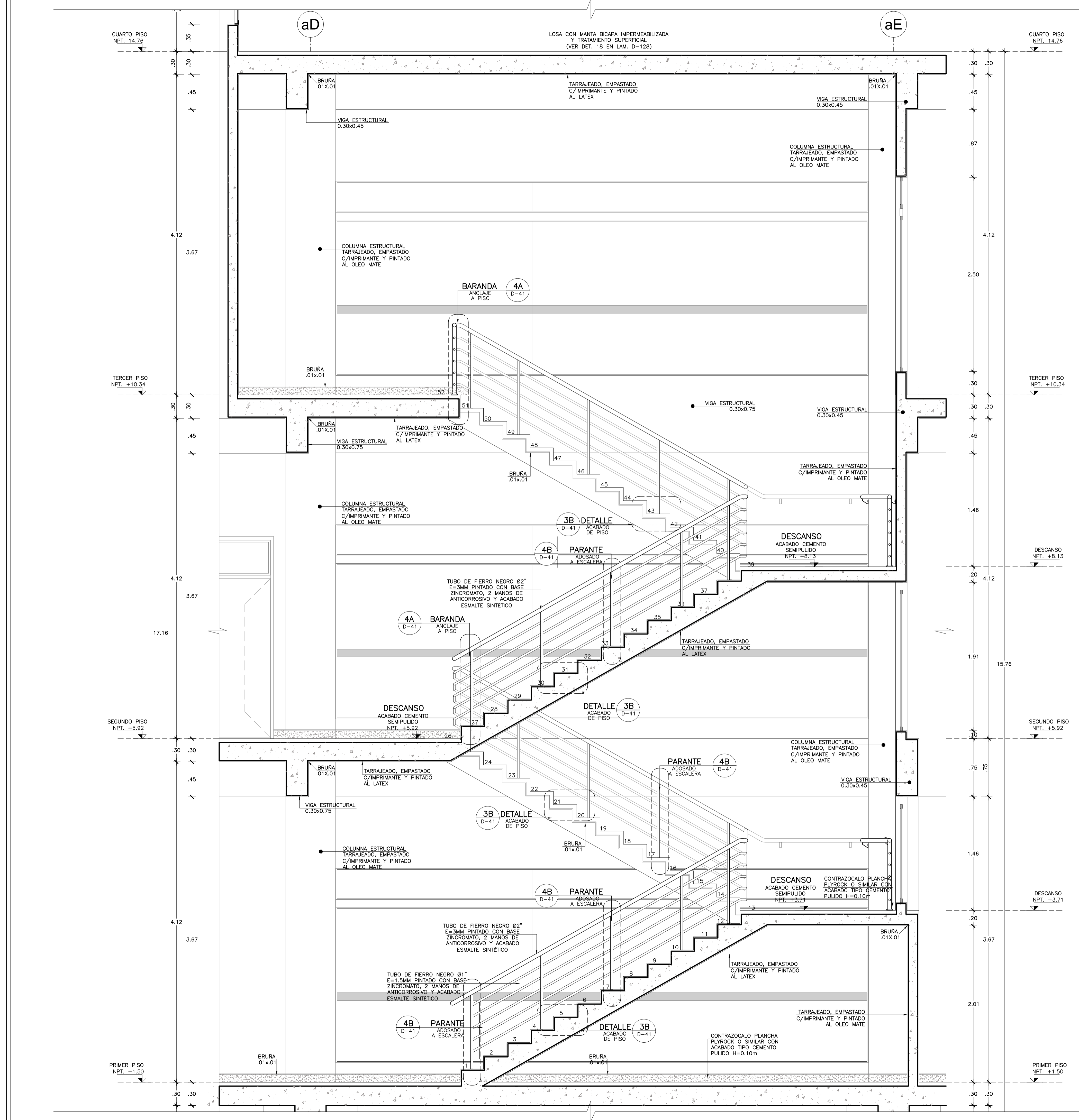
ESCALERA INTEGRADA N° 07 CORTE 1-1 Esc: 1/25
