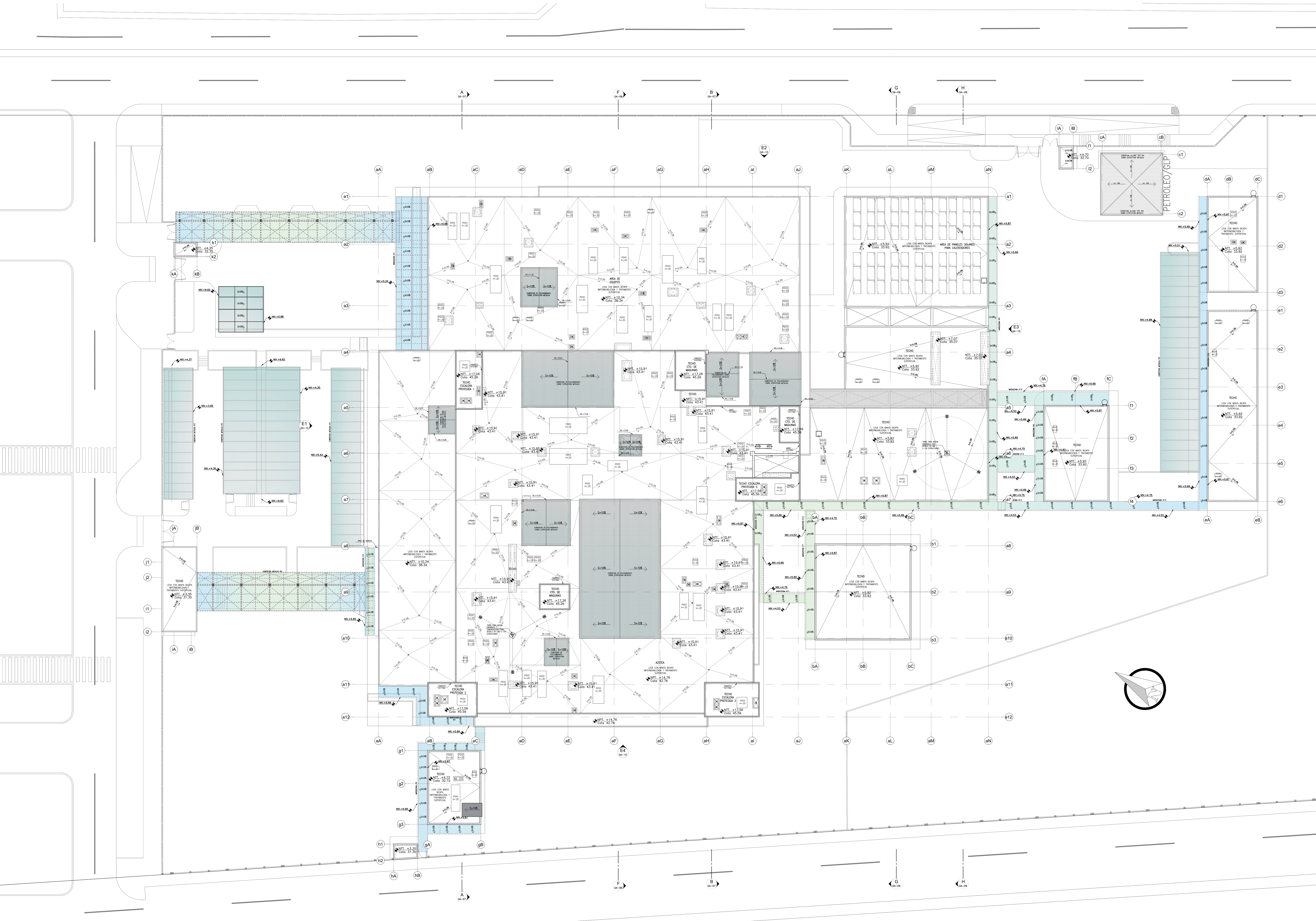
PLANTA TECHOS Esc. 1:200
