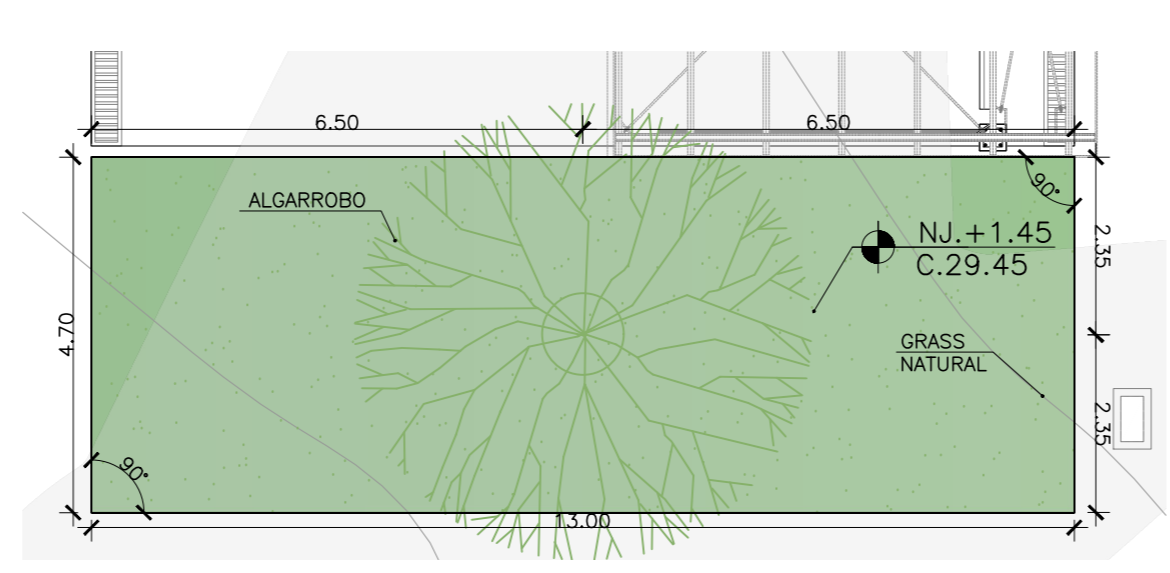
JARDIN N°10 Esc: 1/100
