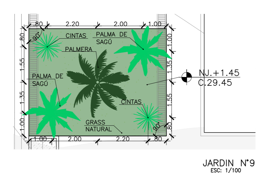
JARDIN N°9 Esc: 1/100
