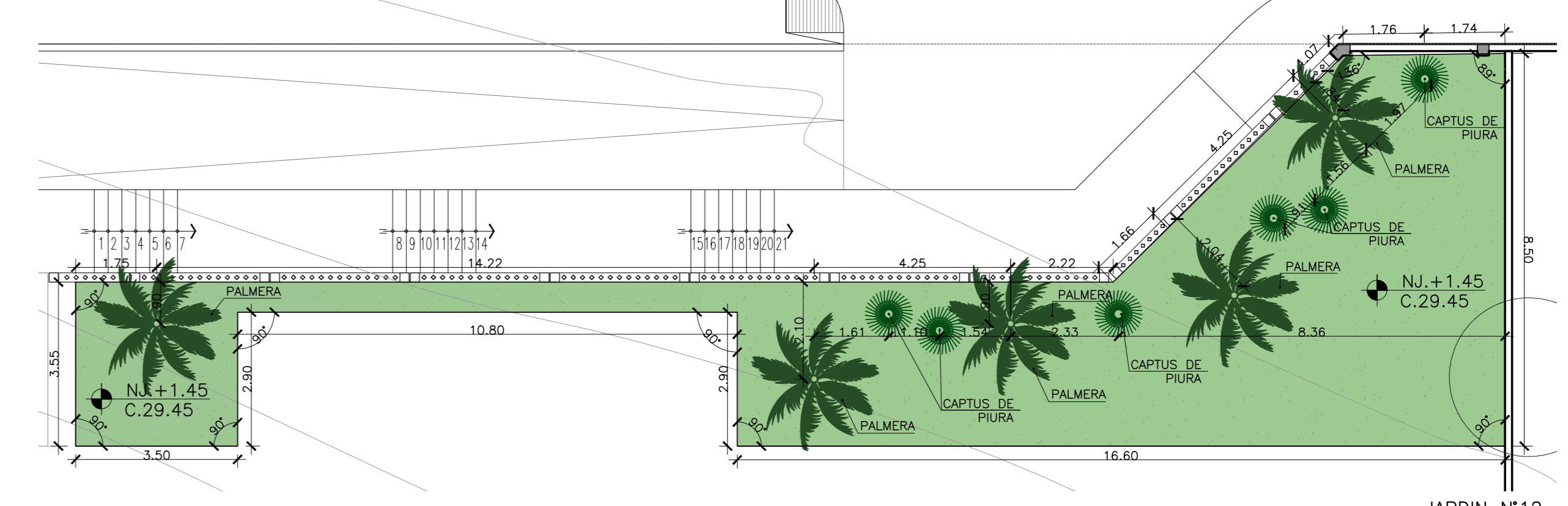
JARDIN N°12 Esc: 1/100
