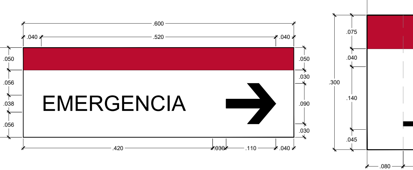
SI-03 INDICATIVO DE PASADIZOS PARA UPSS HOSPITALIZACIÓN ESC. 1/5
