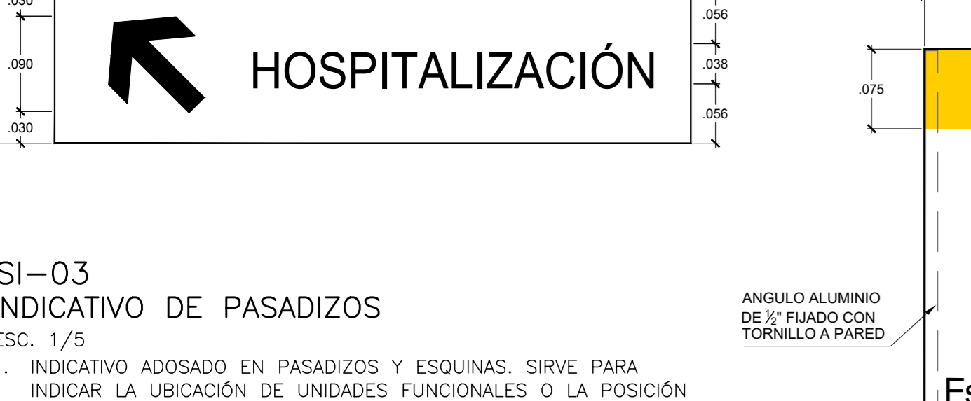
SI-03 INDICATIVO DE PASADIZOS ESC. 1/5
