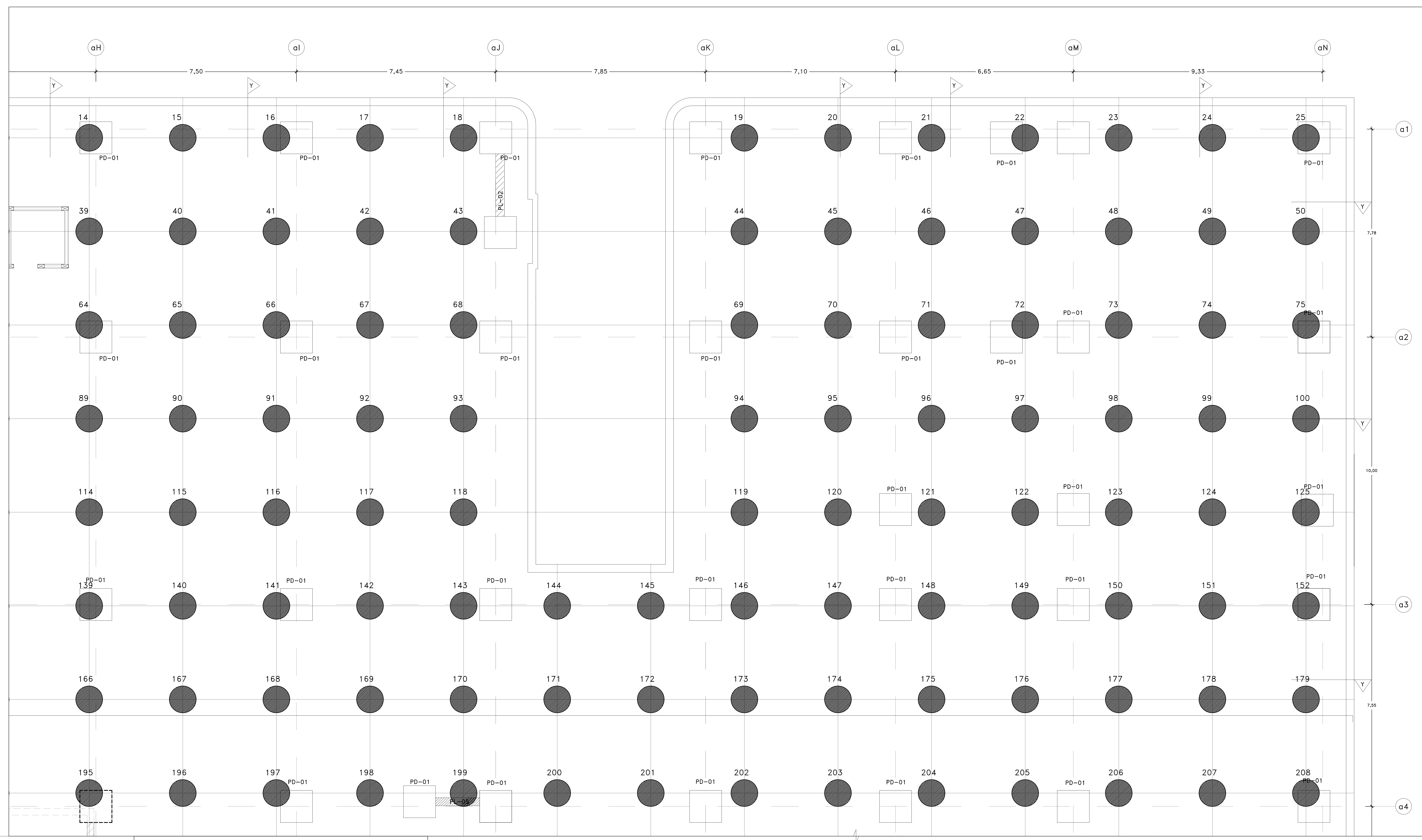
PLANTA DE PILOTES Esc:1/50
