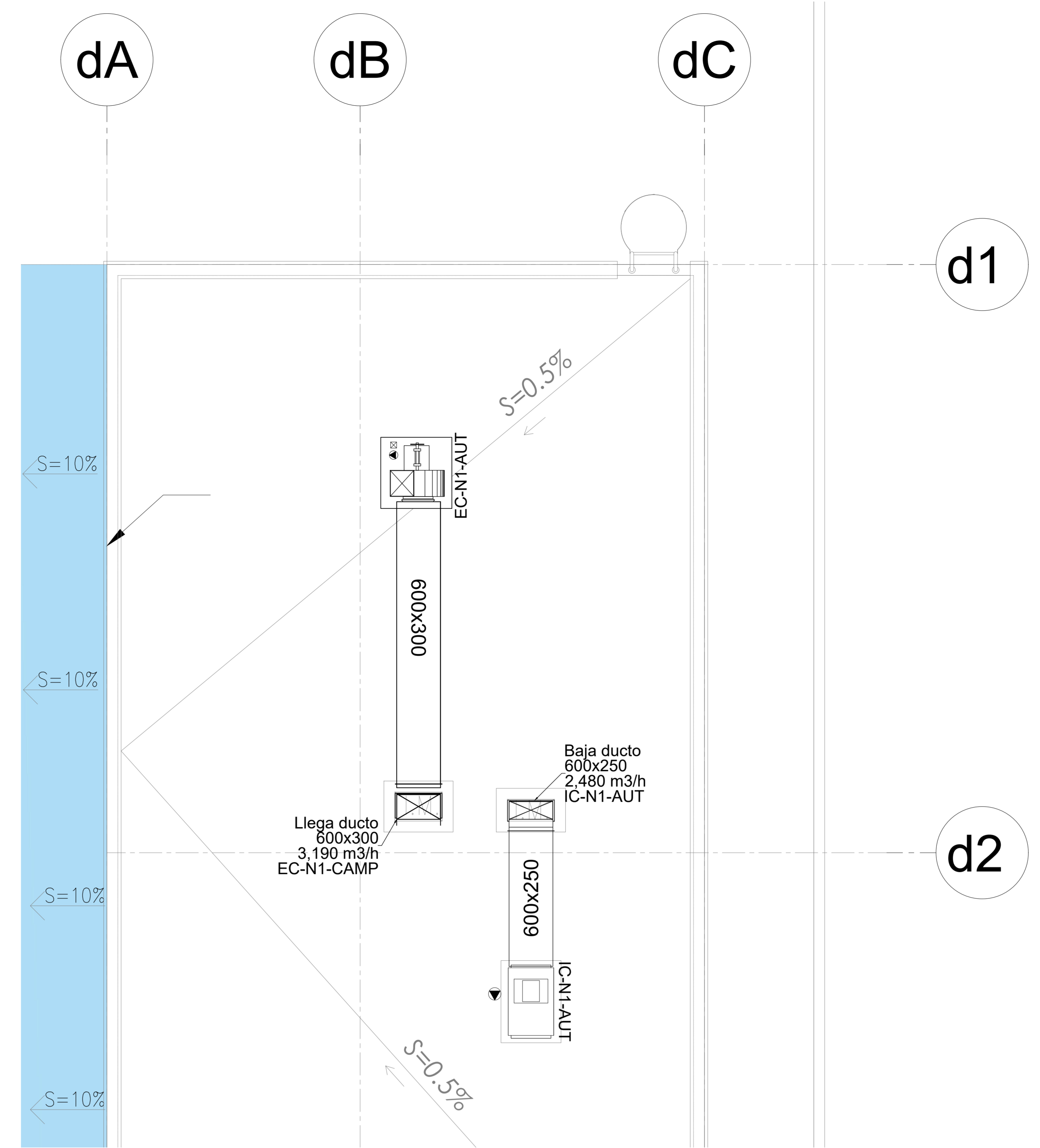
PLANTA TECHO - BLOQUE D ESC: 1/50
