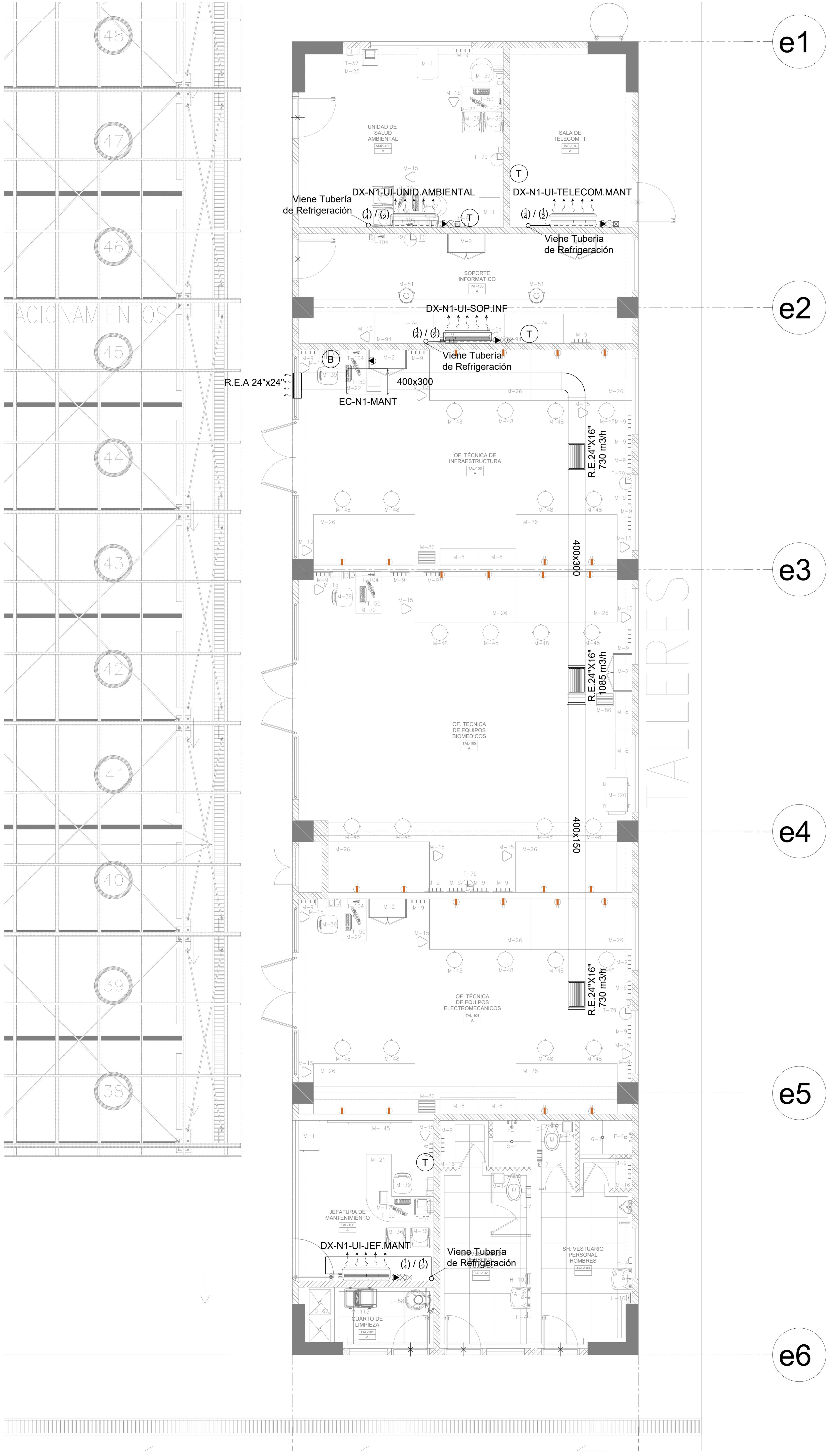
PLANTA PRIMER NIVEL - BLOQUE E ESC: 1/50
