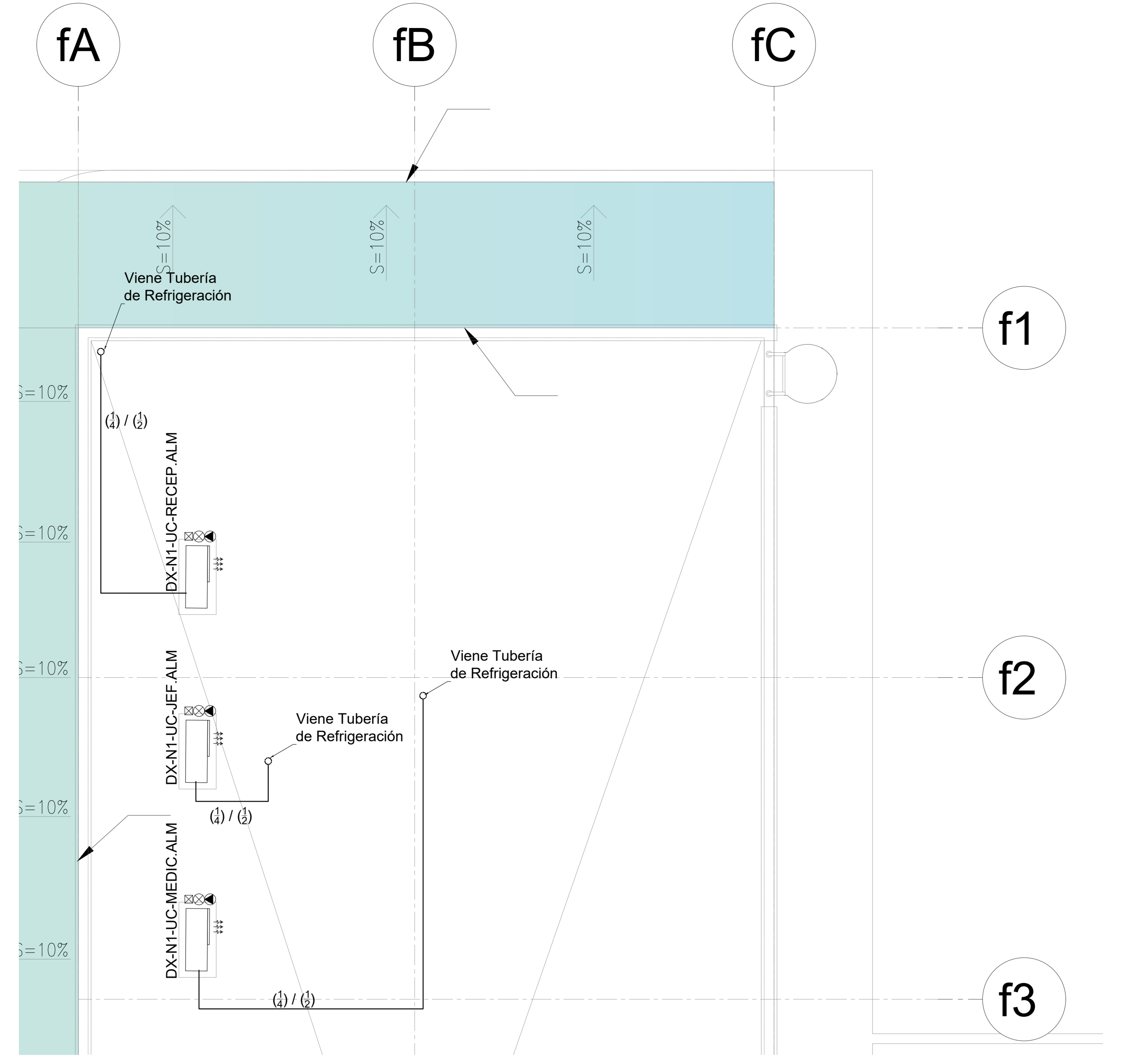
PLANTA TECHO - BLOQUE F ESC: 1/50
