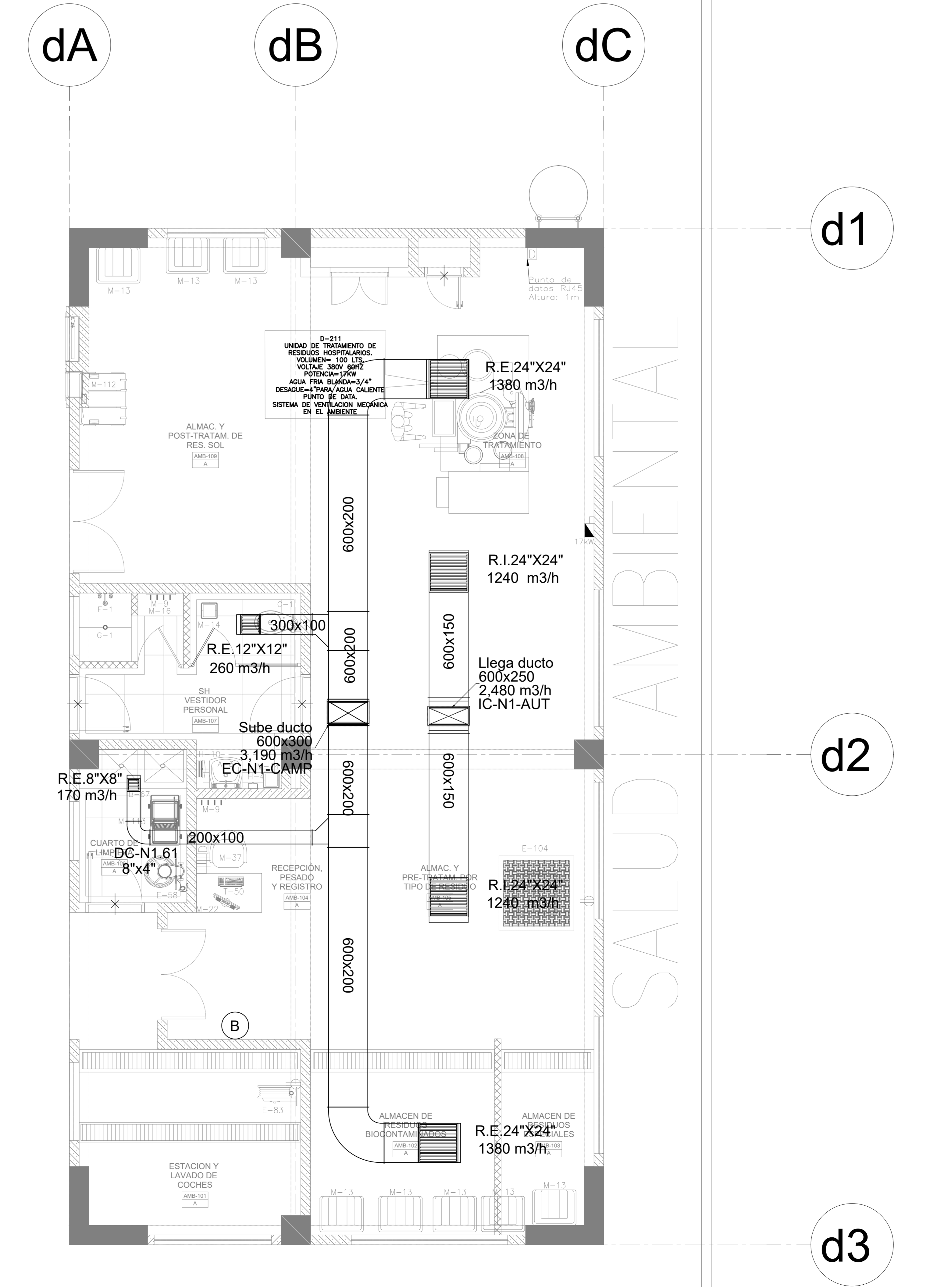
PLANTA PRIMER NIVEL - BLOQUE D ESC: 1/50
