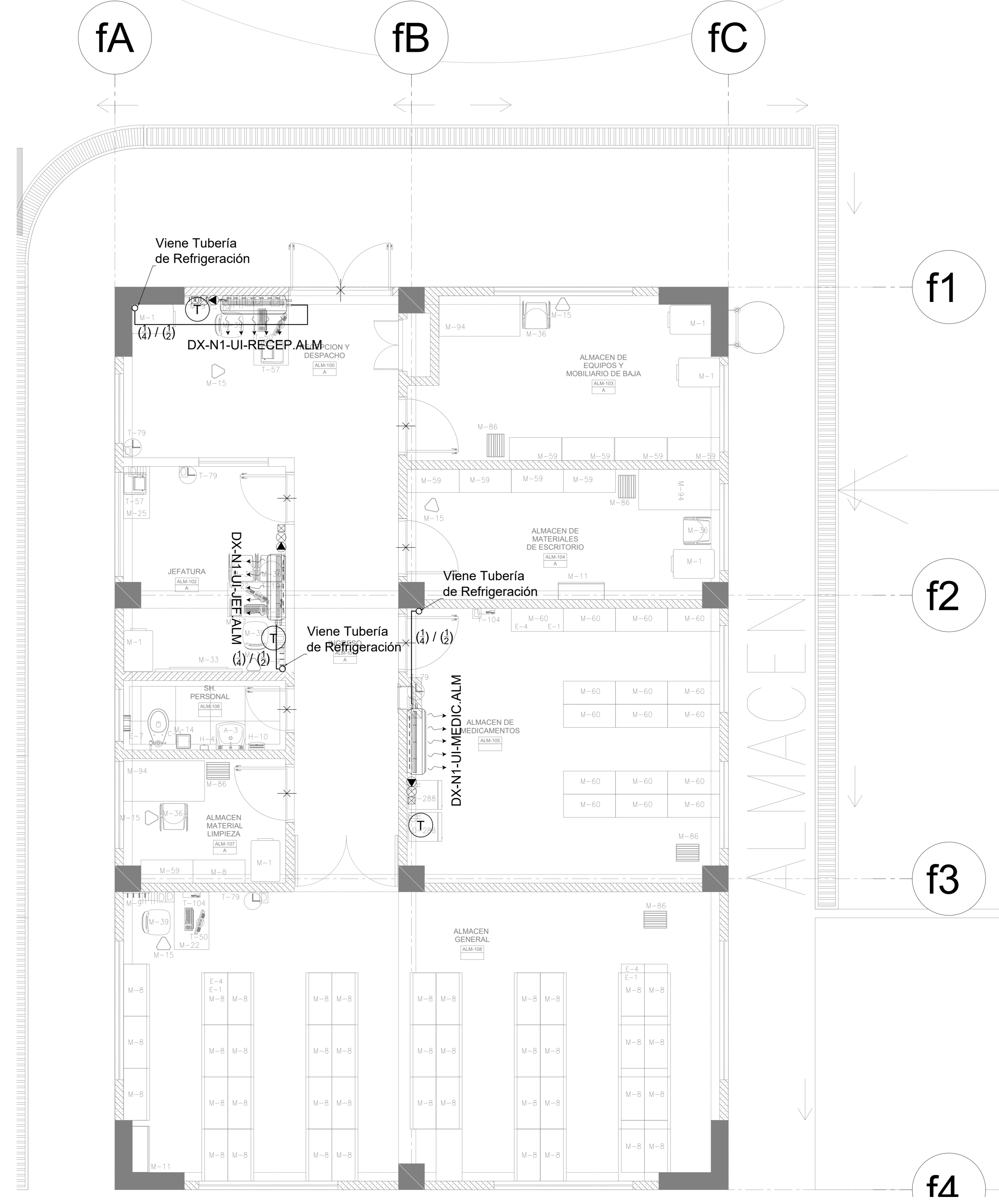
PLANTA PRIMER NIVEL - BLOQUE F ESC: 1/50
