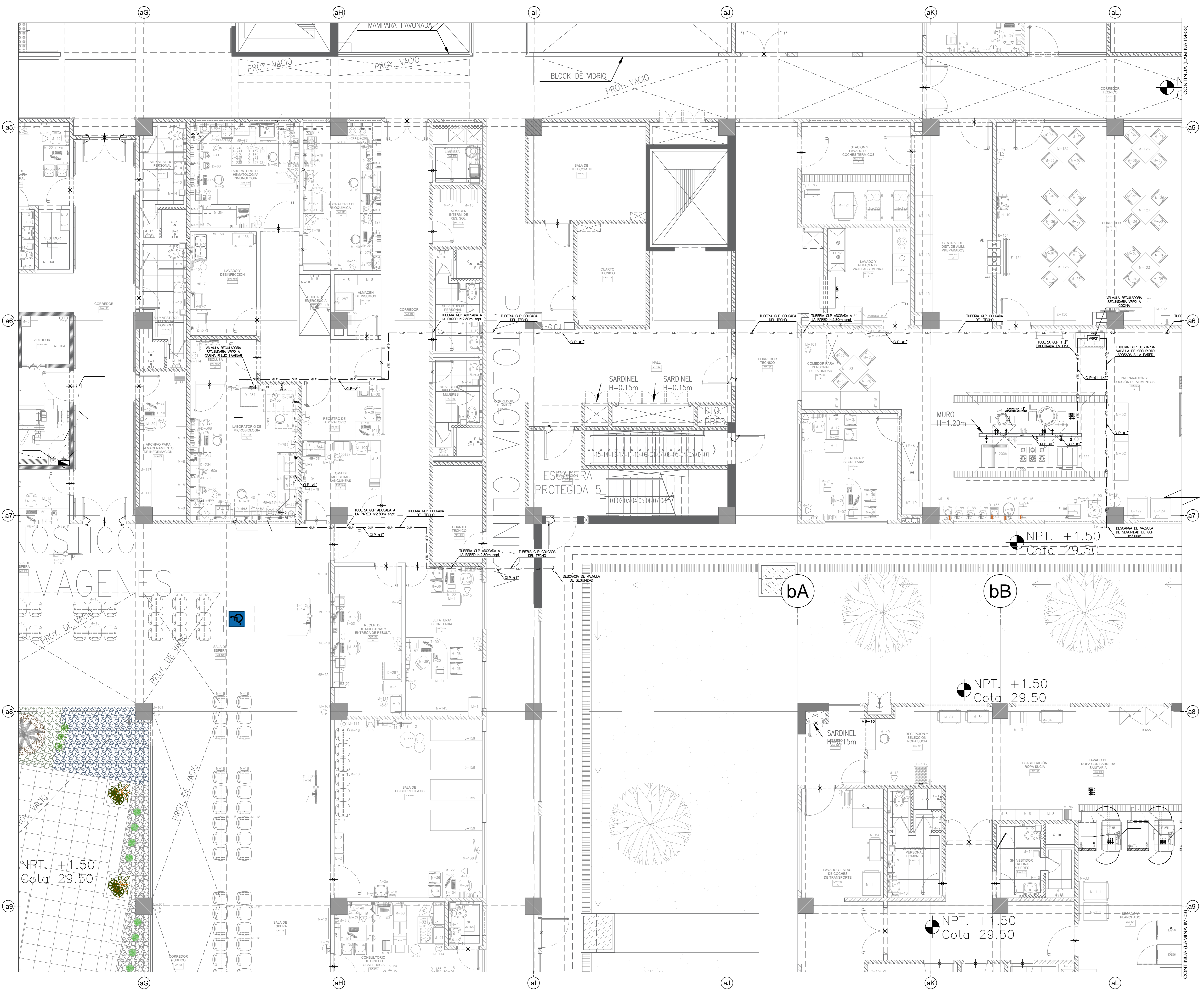
PRIMER PISO Esc. 1/50
