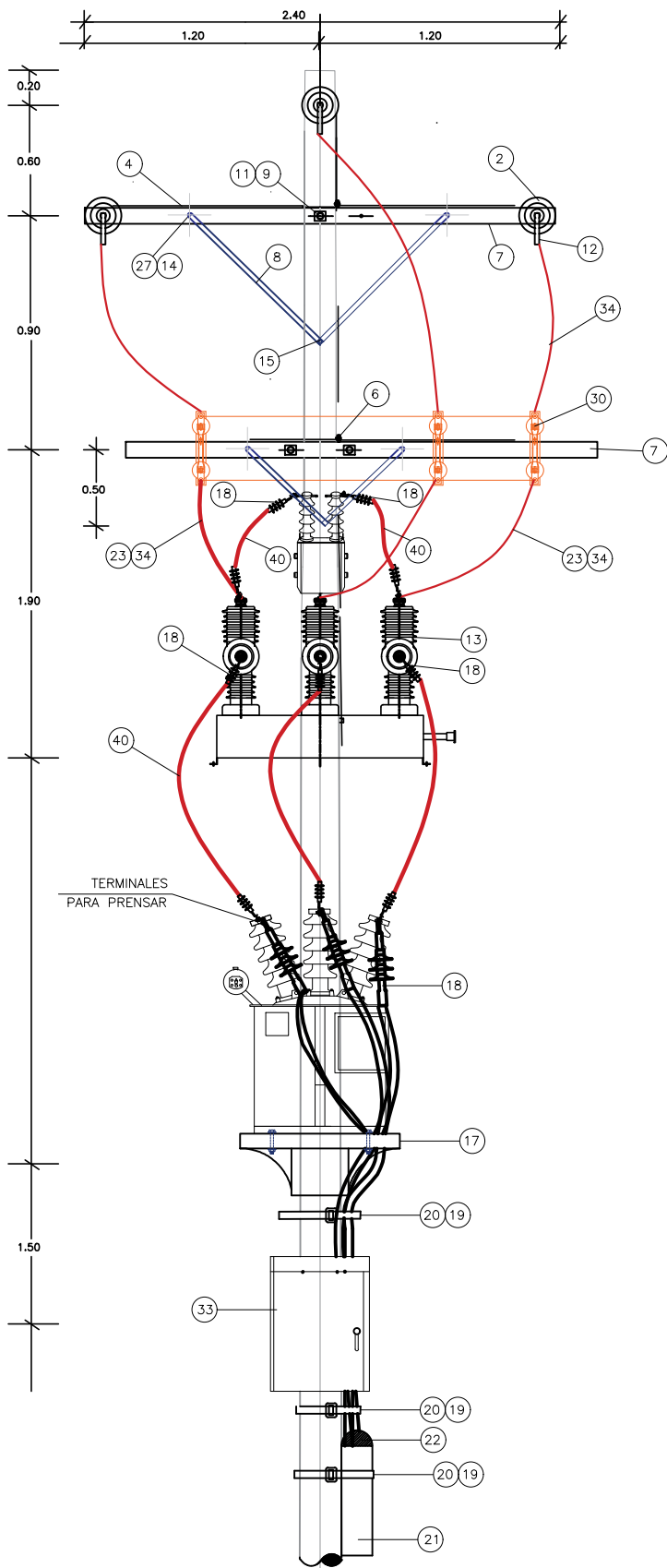
VISTA LATERAL
