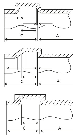
Diseño de ranuras típicas de campanas con juntas de anillo de sello elastomérico.
