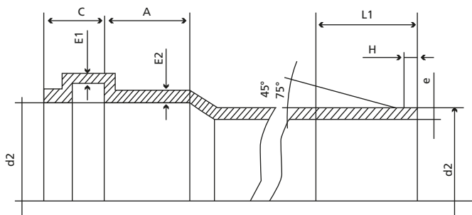
Dimensiones básicas de campanas y espigas para juntas con anillo elastomérico.
